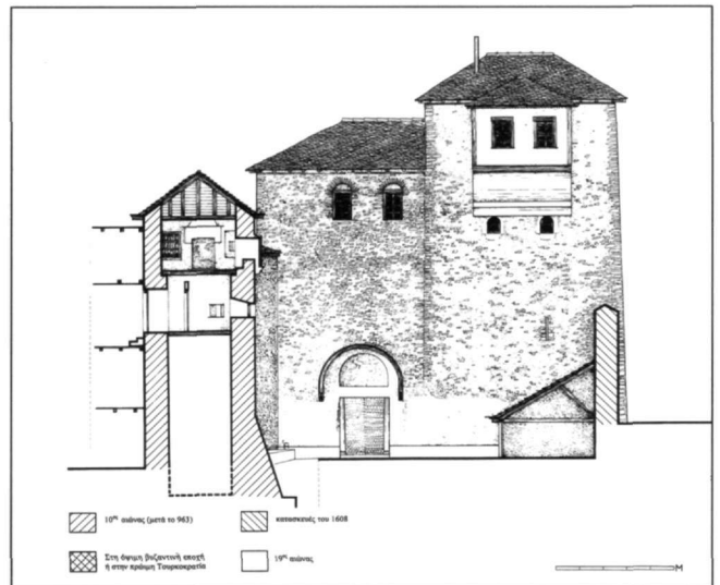
Εικ. 7. Οι δίδυμοι πύργοι της εισόδου πίσω από το προτειχίσμα (τομή ΒΒ).
