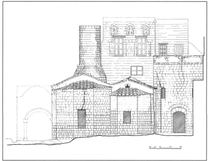
Εικ. 8. Η ανατολική όψη πριν από τις εργασίες αποκατάστασης.
