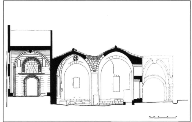
Εικ. 10. Εγκάρσια τομή Α-Α πριν από τις εργασίες αποκατάστασης.
