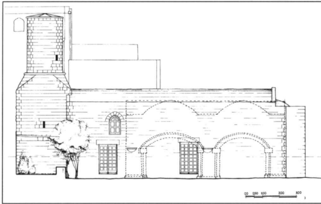
Εικ. 11. Νότια πλευρά. Αποτύπωση.
