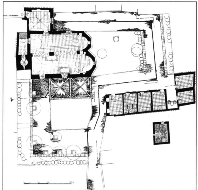
Εικ. 2. Κάτοψη πρότασης αποκατάστασης του ισογείου του μοναστικού συγκροτήματος.
