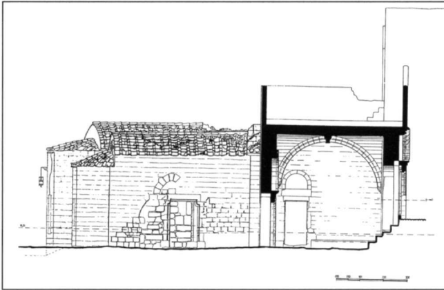
Εικ. 9. Η βόρεια πλευρά πριν από τις εργασίες αποκατάστασης.
