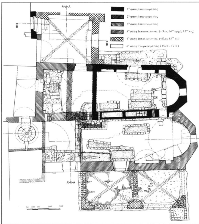
Εικ. 7. Κάτοψη του ισογείου και οι οικοδομικές φάσεις, πριν από τις εργασίες.
