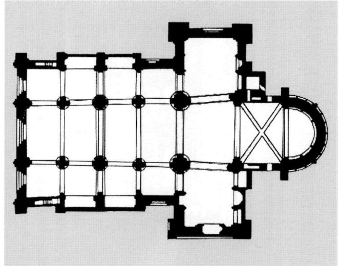
Εικ. 10-11. Η πρόσοψη και η κάτοψη του ναού του Αγίου Μιχαήλ στην Παβία.
