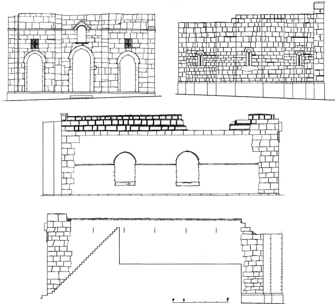
Εικ. 6. Οι σωζόμενοι τοίχοι των πλευρών του καθολικού κατά το 1670.
