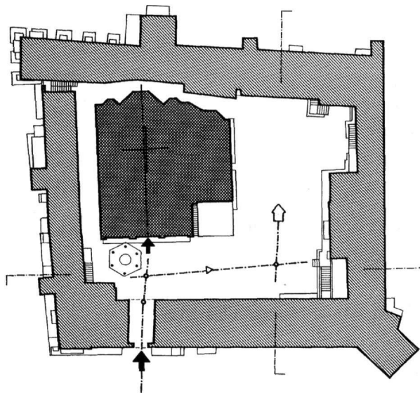
Εικ. 2. Κάτοψη του ισογείου της μονής.
