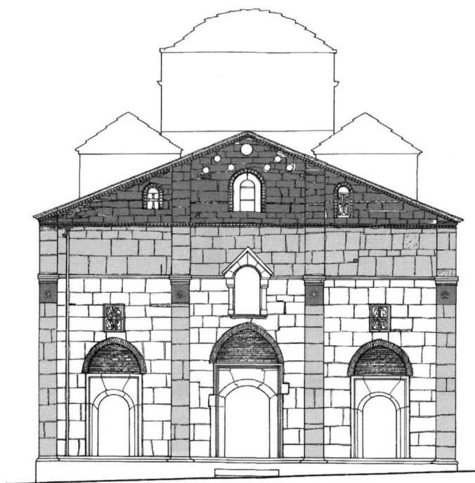
Εικ. 9. Προσπάθεια διαμόρφωσης μιας τετράστυλης πρόσοψης κλασικού ναού στην ανοικοδόμηση του 18ου αιώνα.
