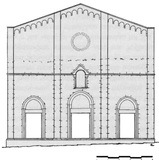
Εικ. 14. Αναπαράσταση της δυτικής πλευράς του λατινικού ναού.
