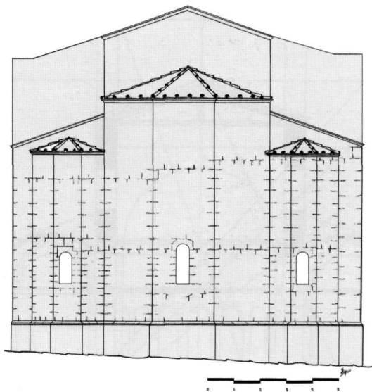
Εικ. 15. Αναπαράσταση της ανατολικής πλευράς του λατινικού ναού.
