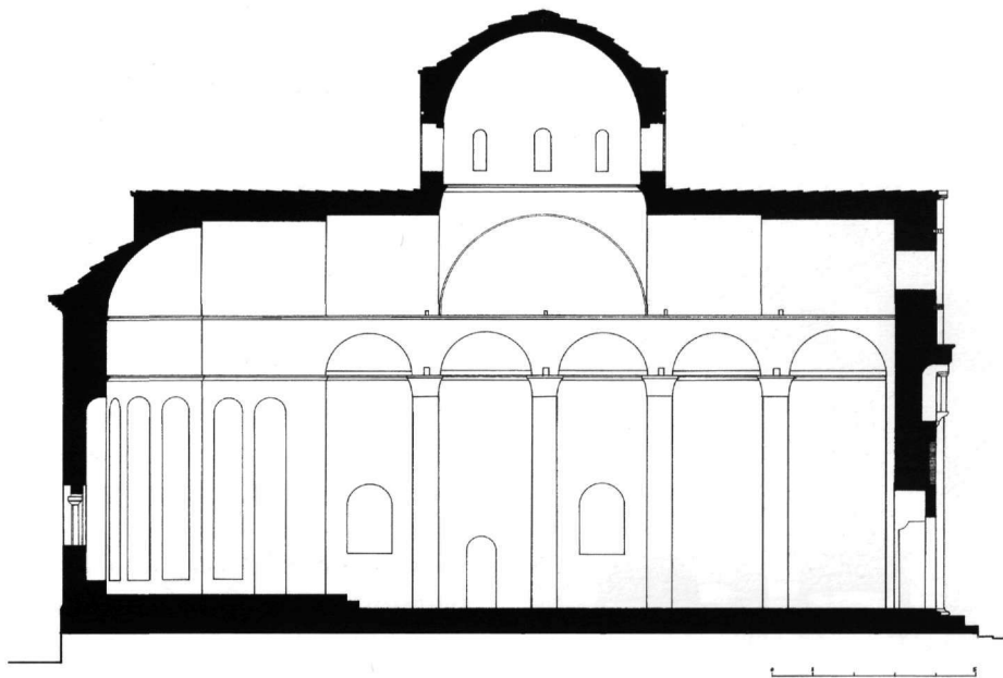
Εικ. 8. Διαμήκης τομή του καθολικού.
