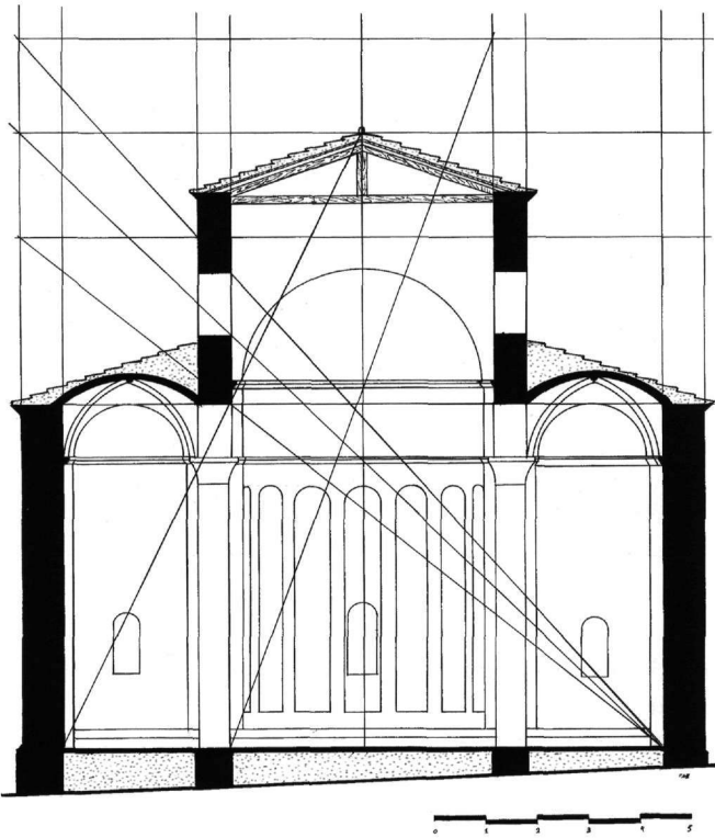
Εικ. 13. Αναπαράσταση της κατά πλάτος τομής του λατινικού ναού της Φανερωμένης.
