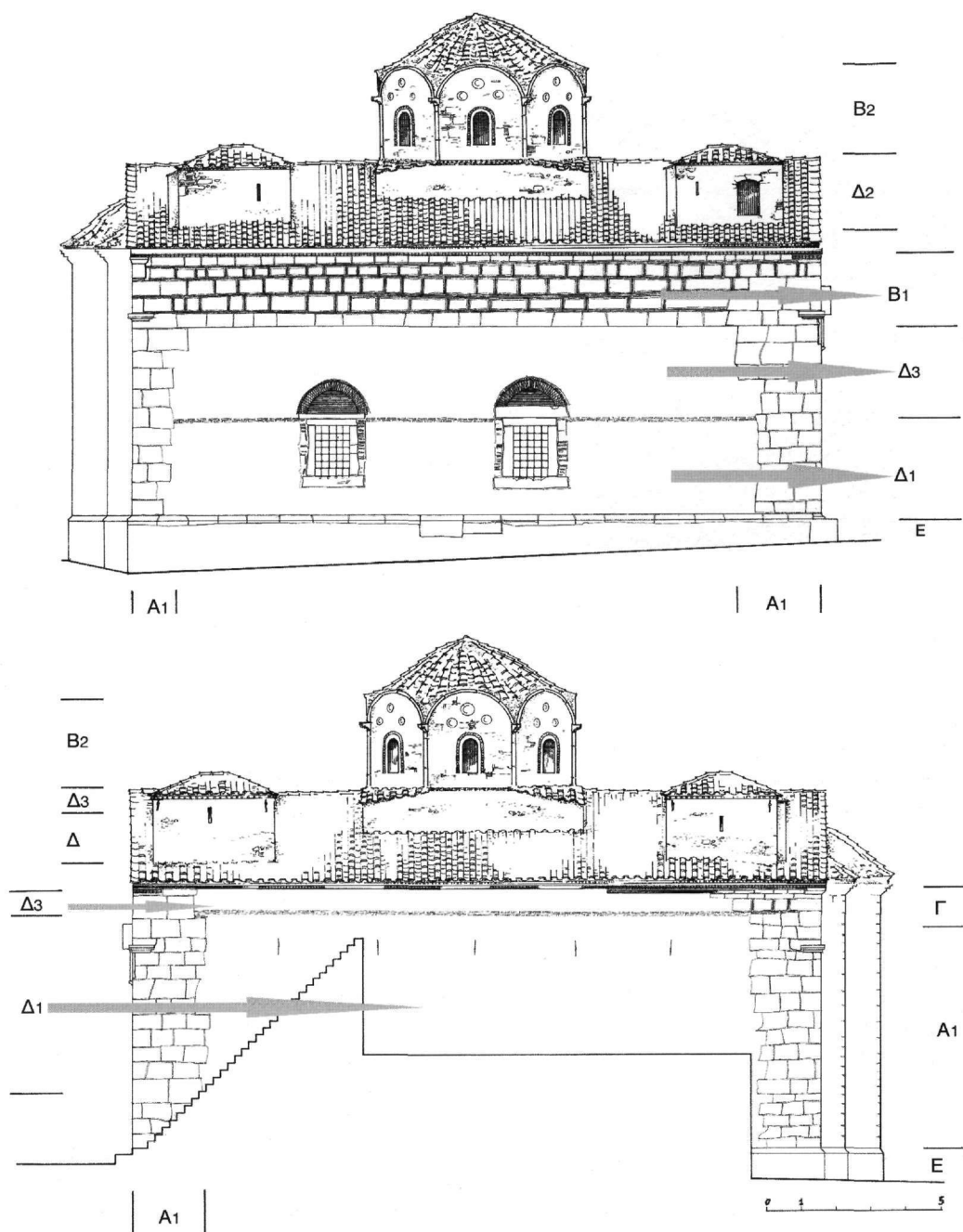
Εικ. 4. Η δόμηση της βορεινής και της νότιας πλευράς του καθολικού.
