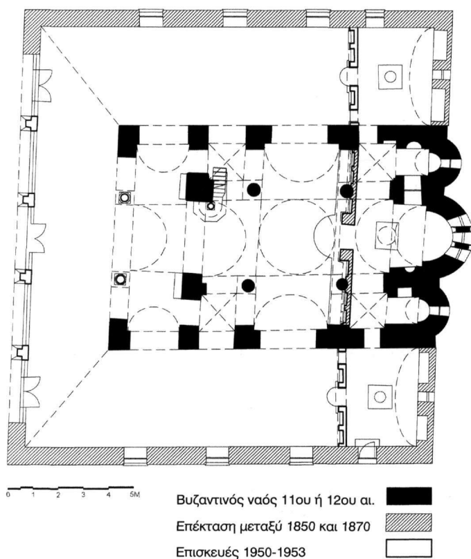
Εικ. 1. Κάτοψη (ανασχεδίαση Ι. Καράνη από σχέδιο αποτύπωσης του Στ. Μαμαλούκου).
