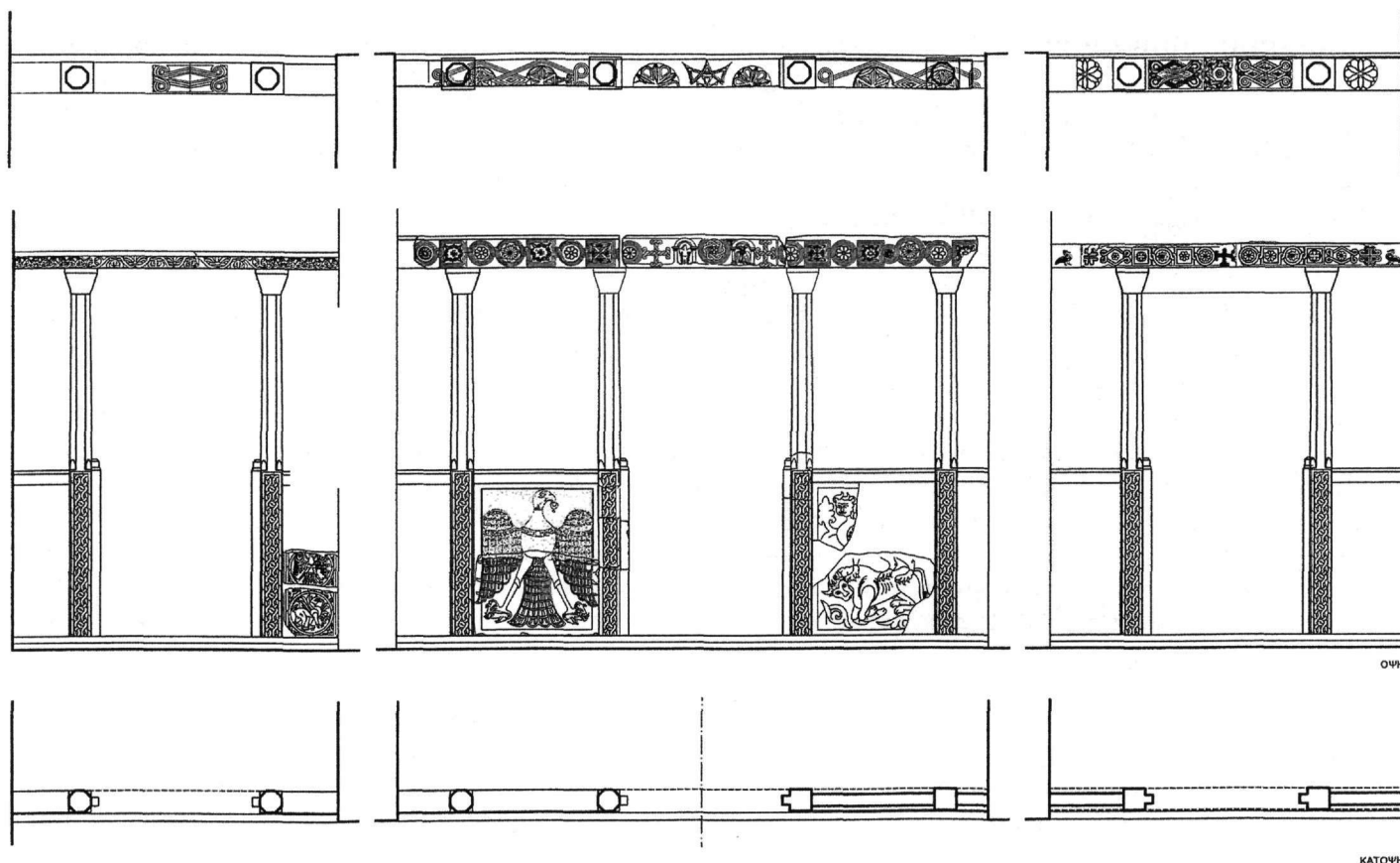
Εικ. 12. Αγία Θεοδώρα Άρτας. Γραφική αναπαράσταση του κεντρικού τμήματος του τέμπλου και των παραβημάτων. Νέα πρόταση.
