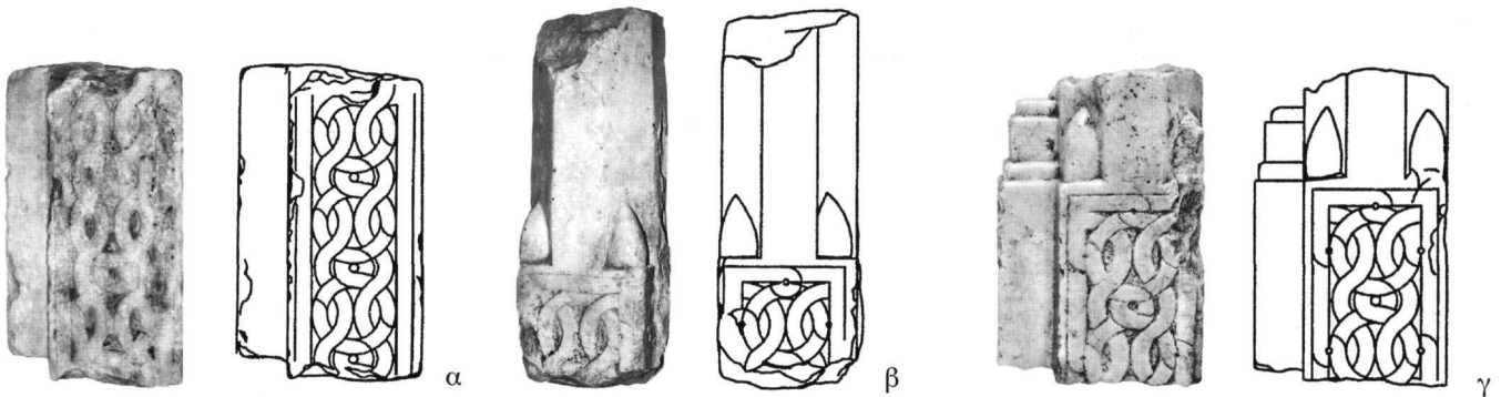
Εἰκ. 7. Πεσσίσκοι αριθ. κατ. 7, 8 και 9.
