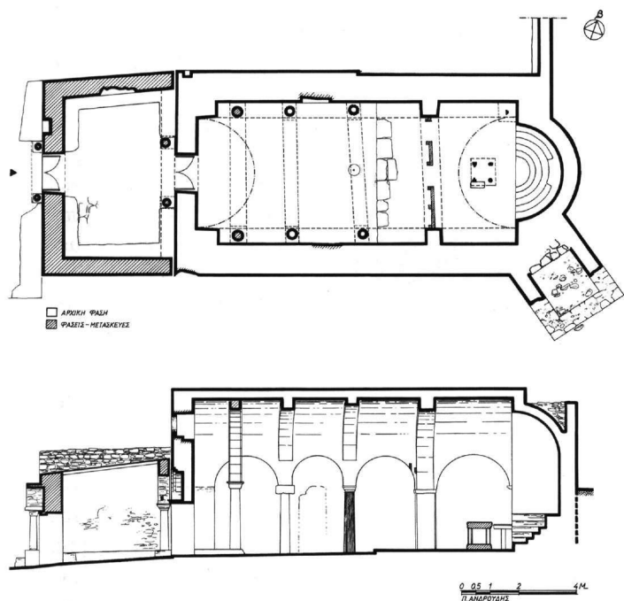
Εικ. 4. Παναγία των Καστριανών. Κάτοψη και κατά μήκος τομή.
