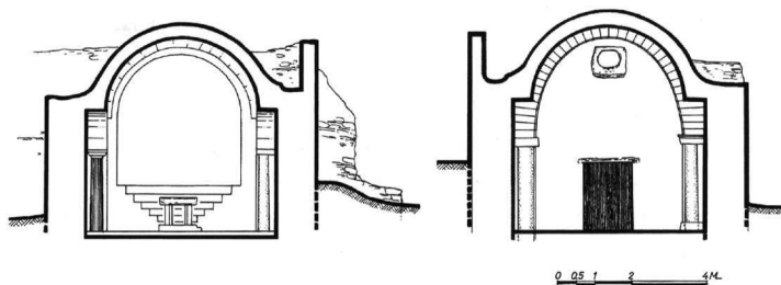
Εικ. 5. Τομή κατά πλάτος και προς το ιερό.
