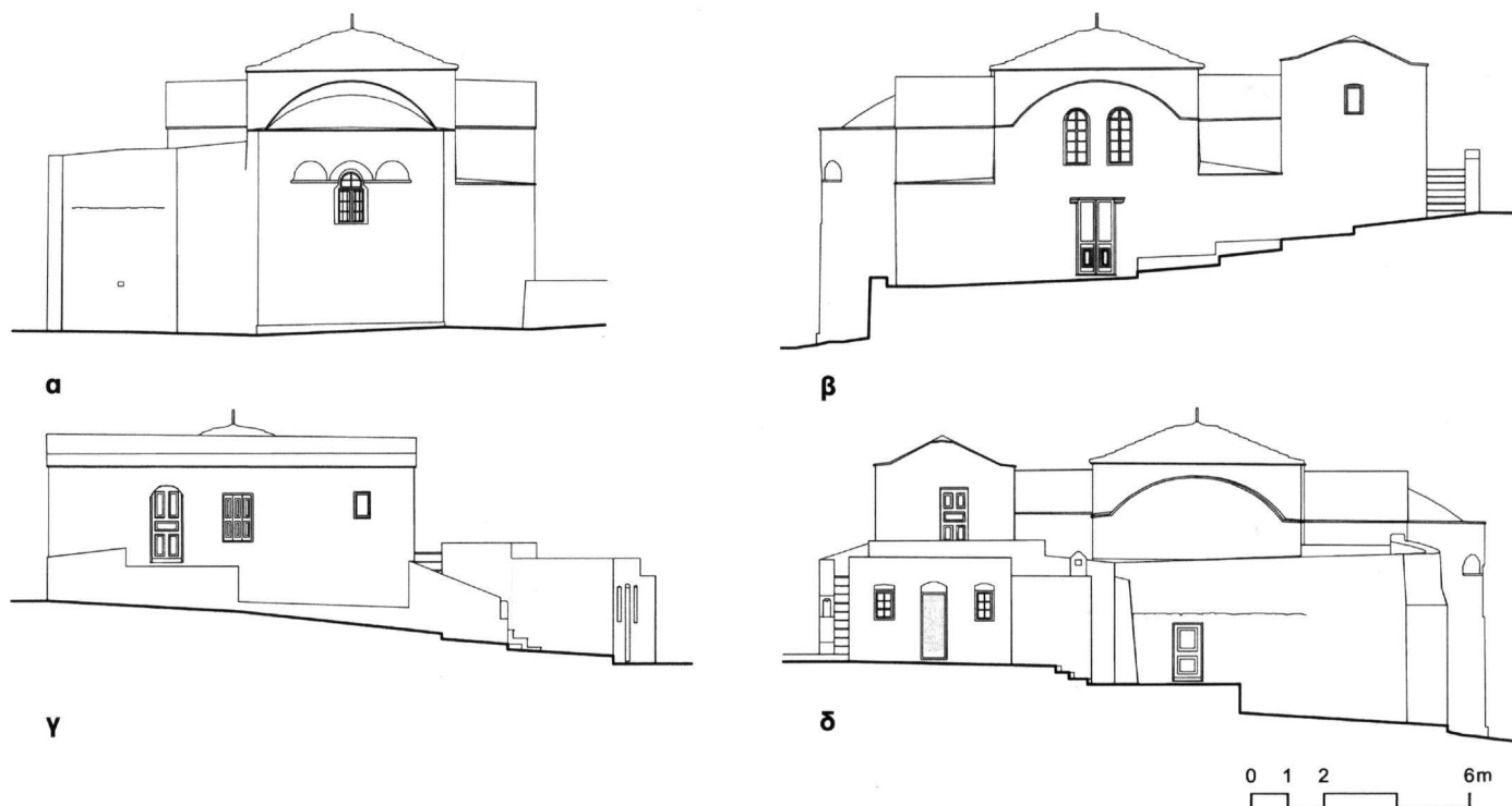
Εικ. 4. Κάλυμνος. Άγιοι Απόστολοι: α. Ανατολική όψη, β. Βόρεια όψη, γ. Δυτική όψη, δ. Νότια όψη.
