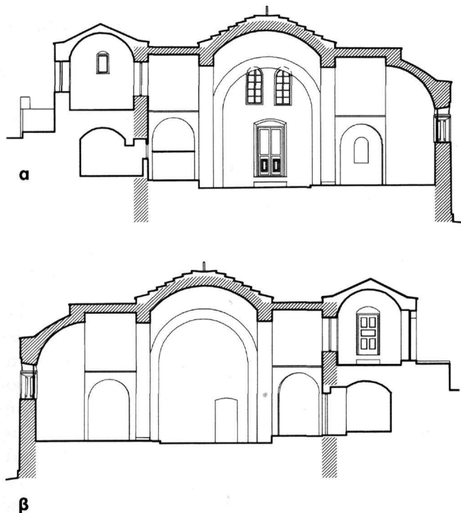
Εικ. 2. Κάλυμνος. Άγιοι Απόστολοι. Τομή κατά μήκος προς Β. και προς Ν.
