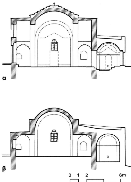
Εικ. 3. Κάλυμνος. Άγιοι Απόστολοι. Τομή κατά πλάτος προς Α. και στο ύψος του ανατολικού σταυρικού σκέλους.
