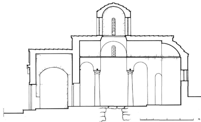
Εικ. 3. Καθολικό μονής Αστερίου. Τομή κατά μήκος.
