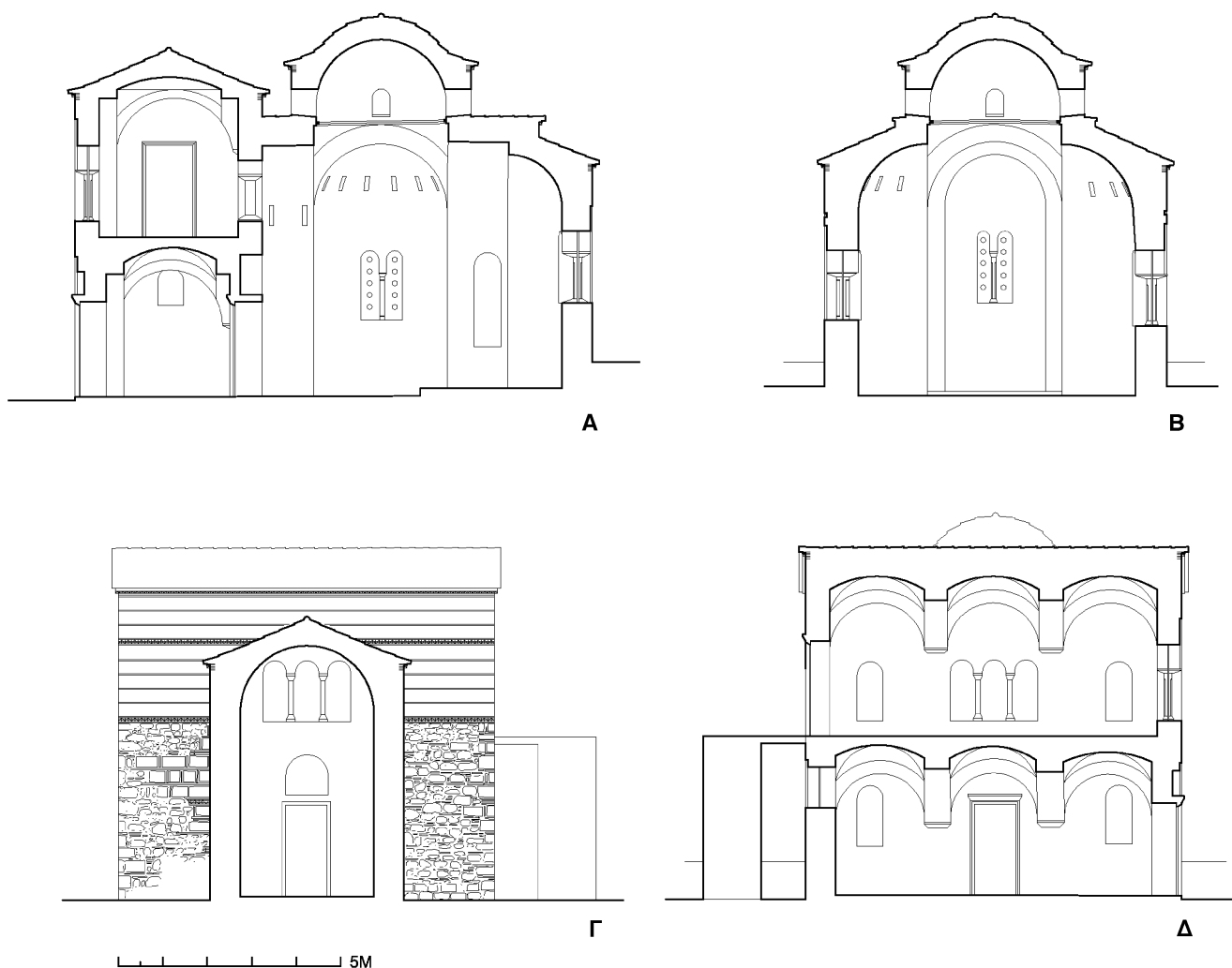
Εικ. 7. Ναός Αγίου Νικολάου. Τομές. Αναπαράσταση (βλ. Εικ. 6): Α. Τομή ΑΑ, Β. Τομή ΒΒ, Γ. Τομή ΓΓ, Δ. Τομή ΔΔ.
