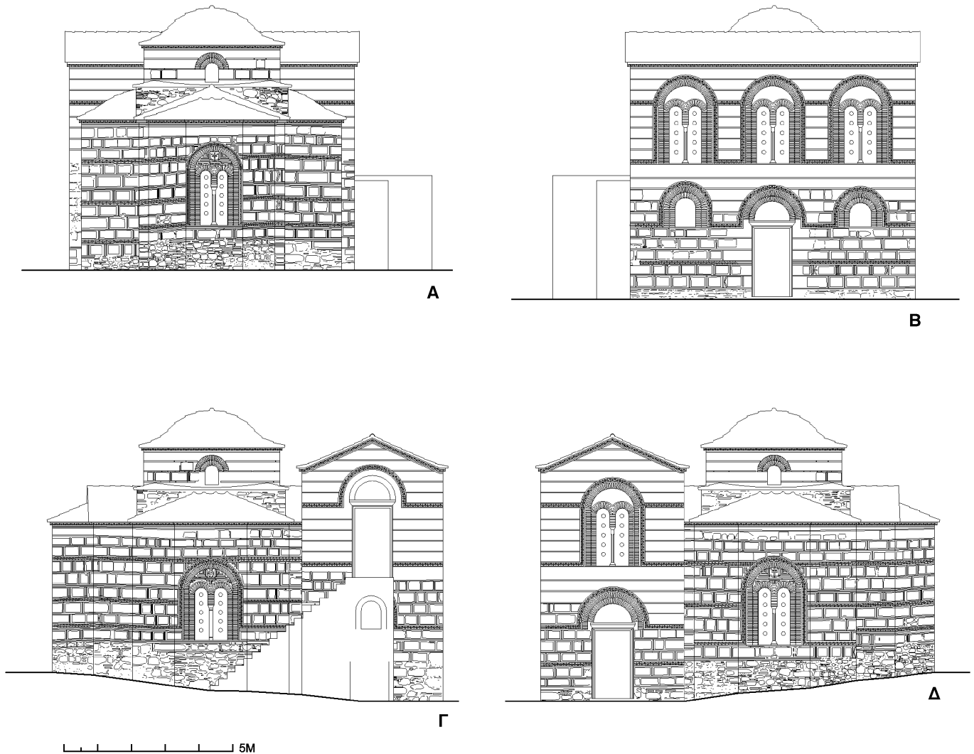
Εικ. 8. Ναός Αγίου Νικολάου. Όψεις. Αναπαράσταση: Α. Ανατολική όψη, Β. Δυτική όψη, Γ. Νότια όψη, Δ. Βόρεια όψη.
