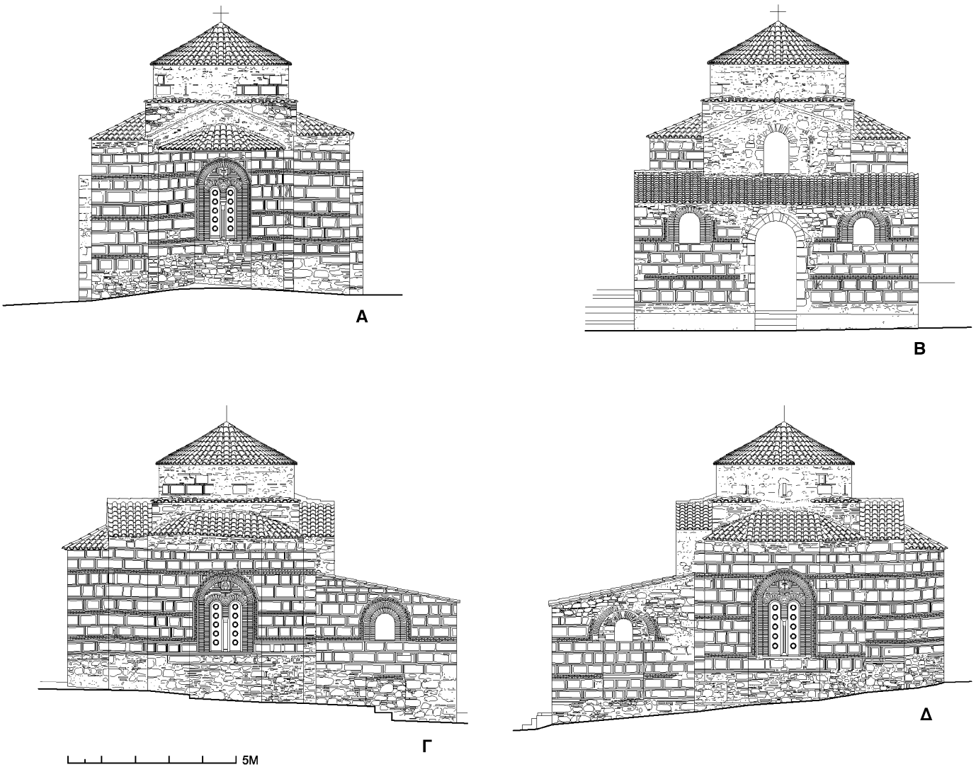
Εικ. 5. Ναός Αγίου Νικολάου. Όψεις. Αποτύπωση με ένδειξη των οικοδομικών φάσεων: Α. Ανατολική όψη, Β. Δυτική όψη, Γ. Νότια όψη, Δ. Βόρεια όψη.
