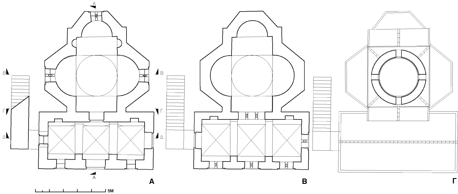
Εικ. 6. Ναός Αγίου Νικολάου. Κατόψεις. Αναπαράσταση: Α. Κάτοψη Α, Β. Κάτοψη Β, Γ. Κάτοψη Γ.
