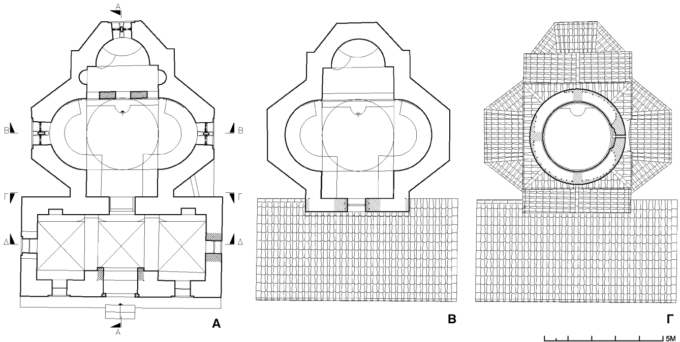
Εικ. 3. Ναός Αγίου Νικολάου. Κατόψεις. Αποτύπωση με ένδειξη των οικοδομικών φάσεων.
