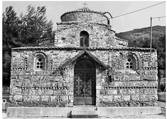
Εικ. 2. Πλατάνι Αχαΐας, Ναός Αγίου Νικολάου. Αποψη από τα δυτικά (Σεπτέμβριος 2005).
