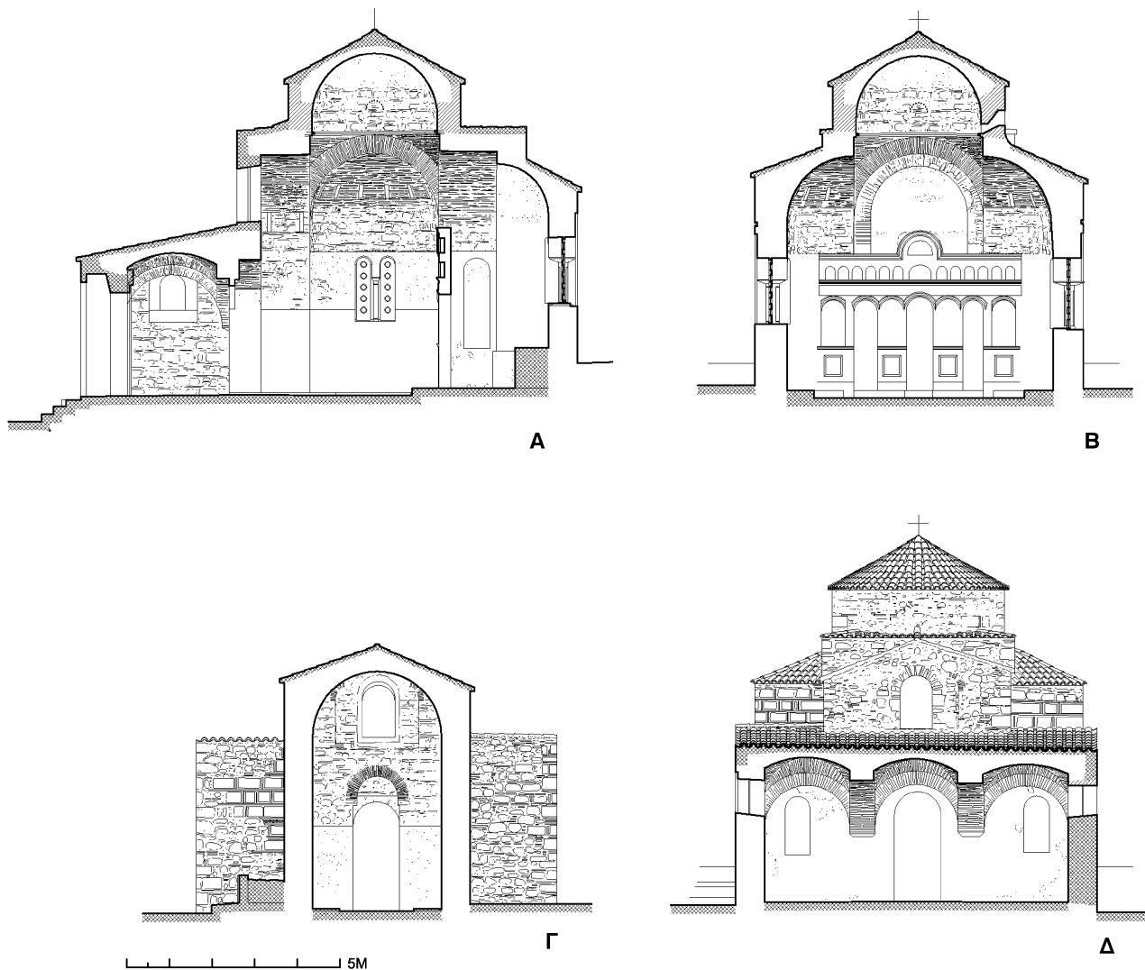
Εικ. 4. Ναός Αγίου Νικολάου. Τομές. Αποτύπωση με ένδειξη των οικοδομικών φάσεων (βλ. Εικ. 3): Α. Τομή ΑΑ, Β. Τομή ΒΒ, Γ. Τομή ΓΓ, Δ. Τομή ΔΔ.
