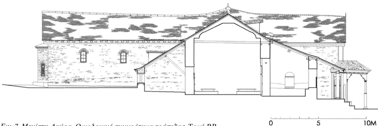
Εικ. 7. Μεγίστη Λαύρα. Οικοδομικό συγκρότημα τράπεζας. Τομή ΒΒ.
