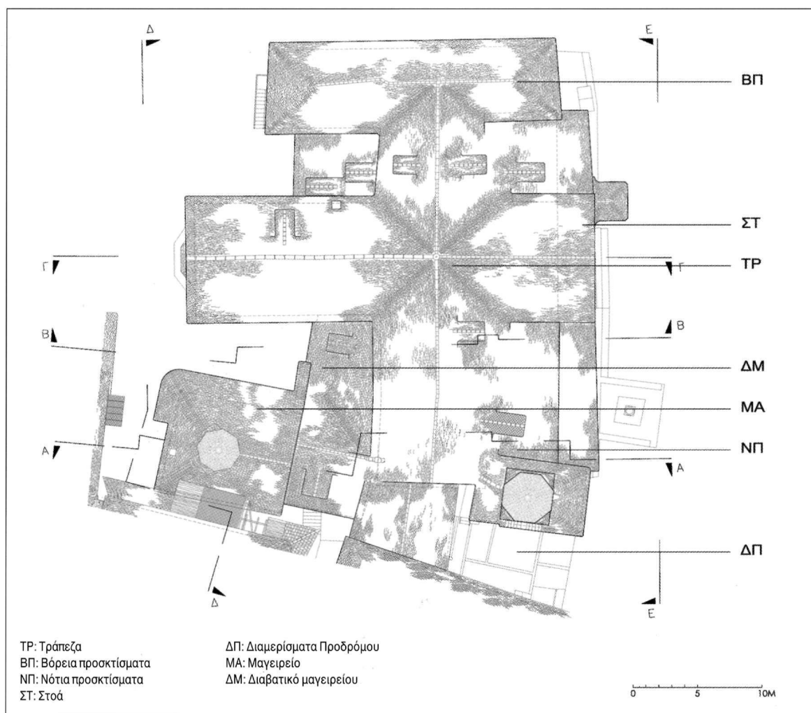
Εικ. 2. Μεγίστη Λαύρα. Οικοδομικό συγκρότημα τράπεζας. Κάτοψη στεγών με ένδειξη των επιμέρους κτηρίων.
