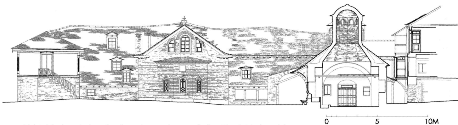
Εικ. 9. Μεγίστη Λαύρα. Οικοδομικό συγκρότημα τράπεζας. Τομή ΔΔ. Δυτική όψη.
