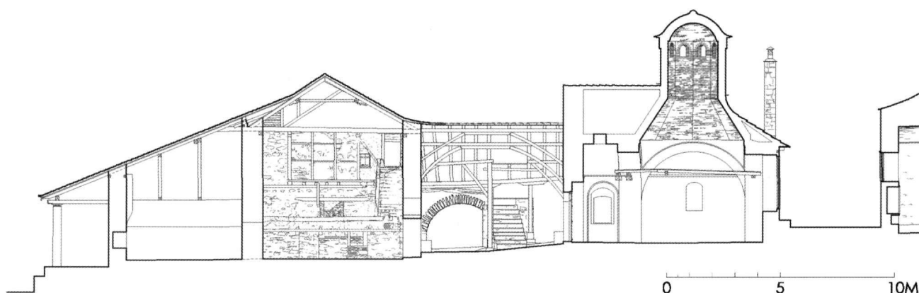
Εικ. 6. Μεγίστη Λαύρα. Οικοδομικό συγκρότημα τράπεζας. Τομή ΑΑ.
