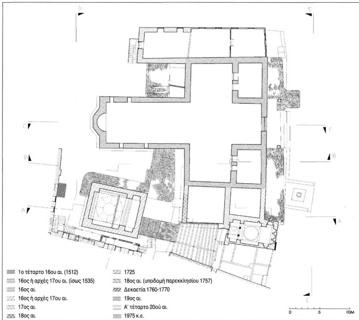
Εικ. 5. Μεγίστη Λαύρα. Οικοδομικό συγκρότημα τράπεζας. Κάτοψη Γ. Οικοδομικές φάσεις.
