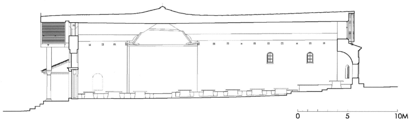
Εικ. 8. Μεγίστη Λαύρα. Οικοδομικό συγκρότημα τράπεζας. Τομή ΓΓ.
