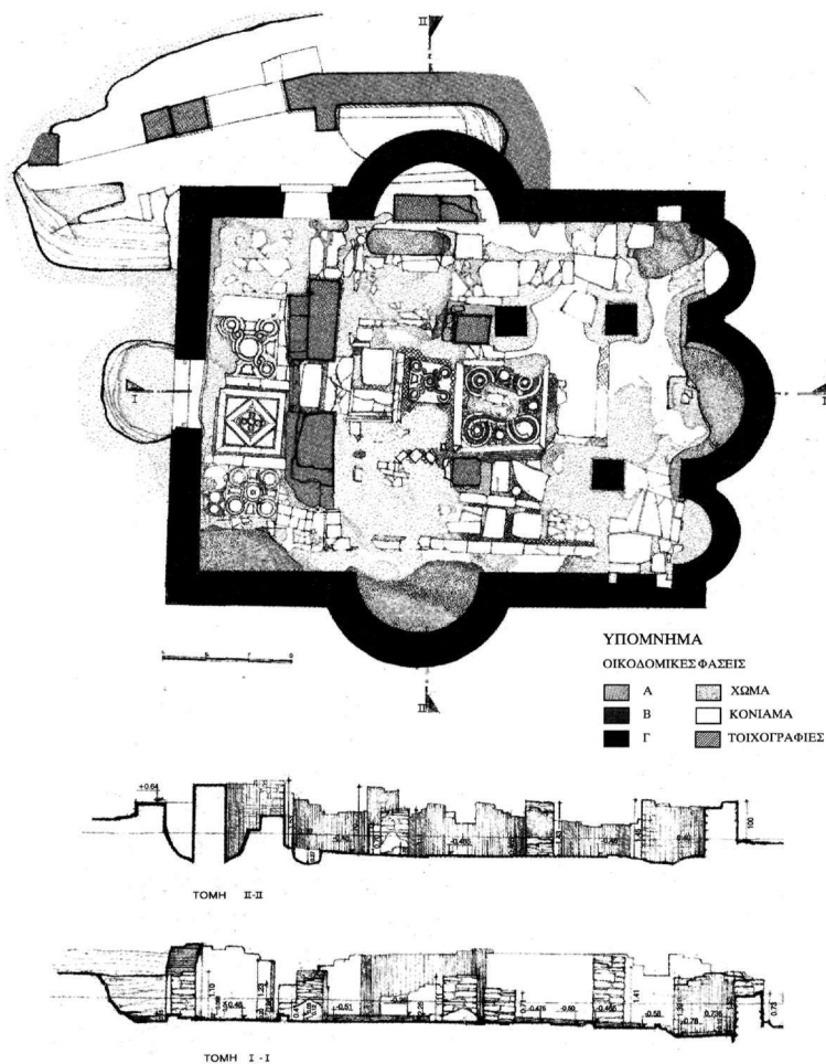
Εικ. 3. Λυκοβουνό. Ανασκαφή της μονής του Αγίου Γεωργίου. Κάτοψη και τομές Ι-Ι, ΙΙ-ΙΙ.
