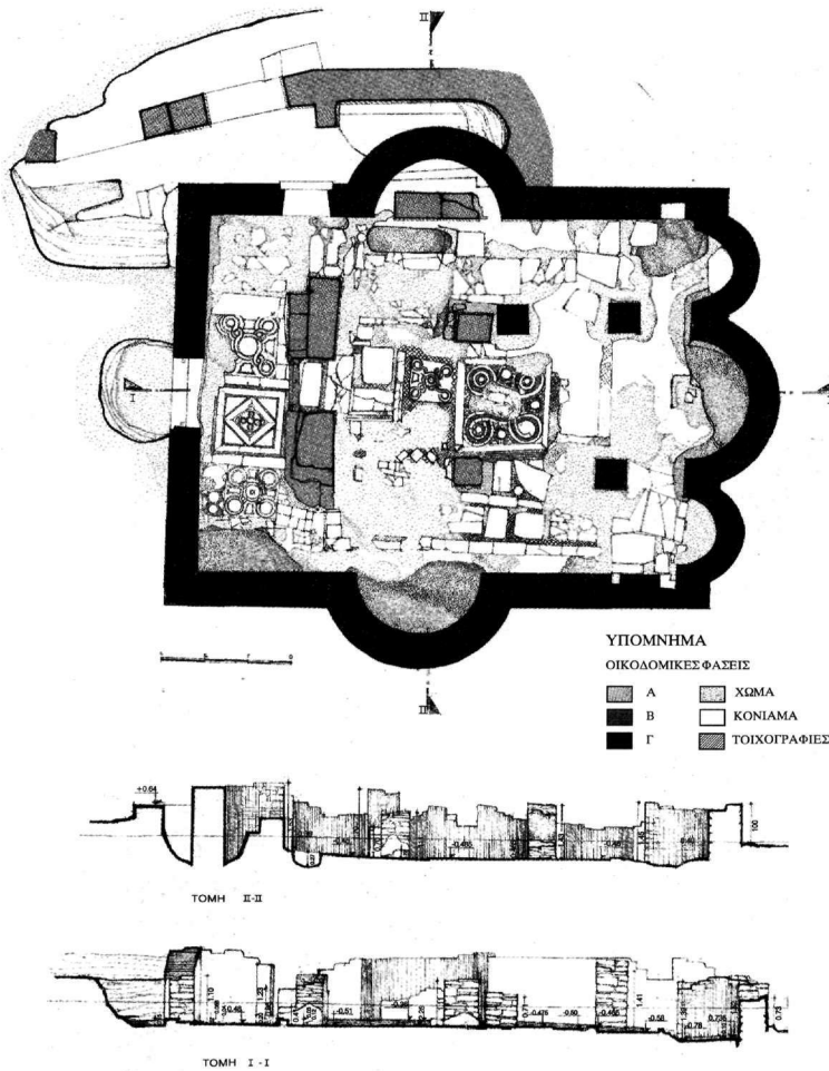
Εικ. 3. Λυκοβουνό. Ανασκαφή της μονής του Αγίου Γεωργίου. Κάτοψη και τομές I-I, II-II.
