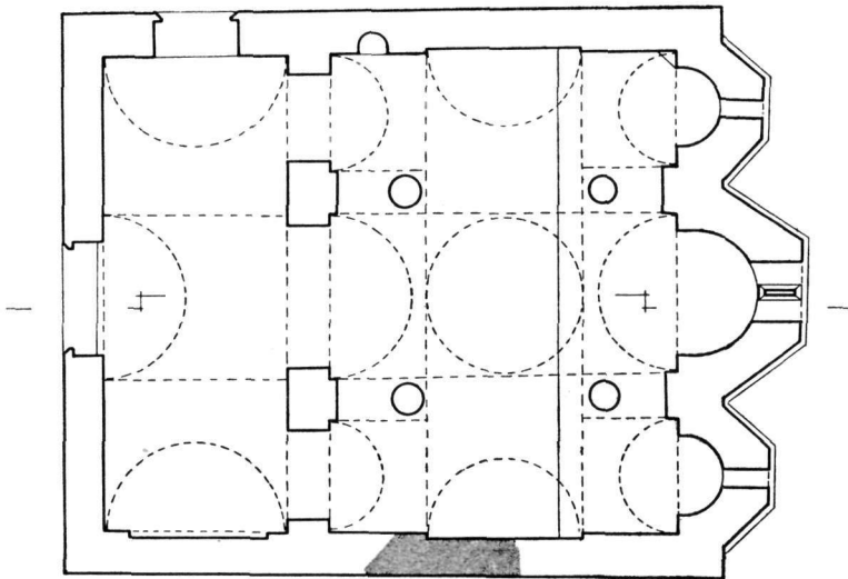
Εἰκ. 5. Ναὸς Ἁγ. Ἀσωμάτων. Κάτοψις καὶ τομὴ κατὰ μῆκος μετὰ τὴν ἀποκατάστασιν.
