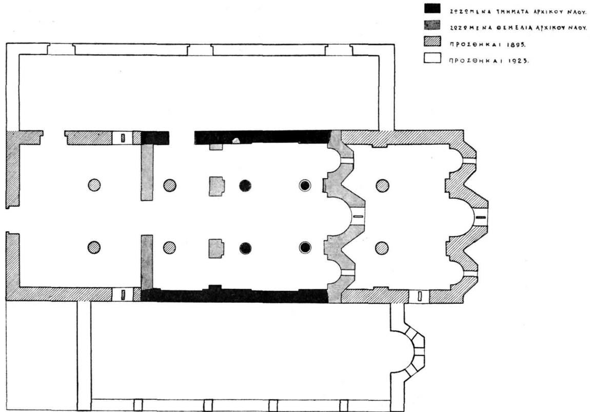
Εἰκ. 1. Ναός Ἀσωμάτων. Κάτωφλι τοῦ μνημείου πρὸ τῶν ἐργασιῶν.
