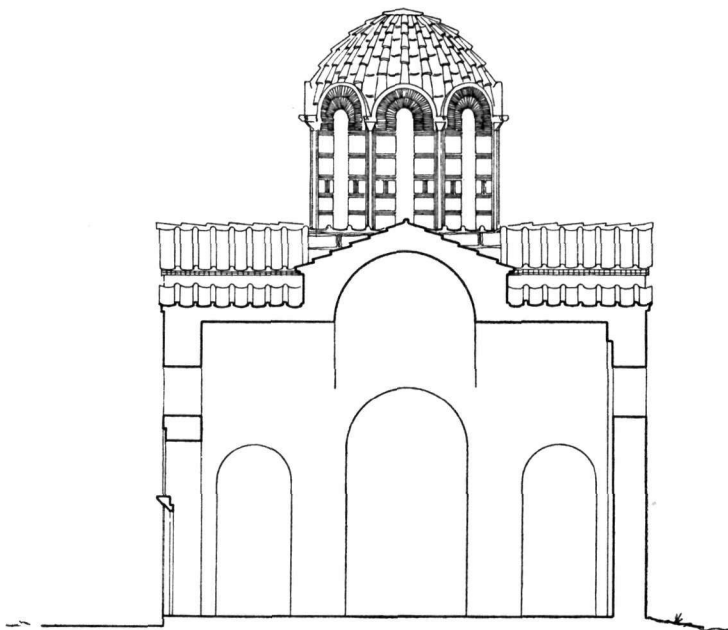
Είχ. 6. Τομή κατά πλάτος του κυρίως ναού και του νάρθηκος μετά την άποκατάστασιν.
