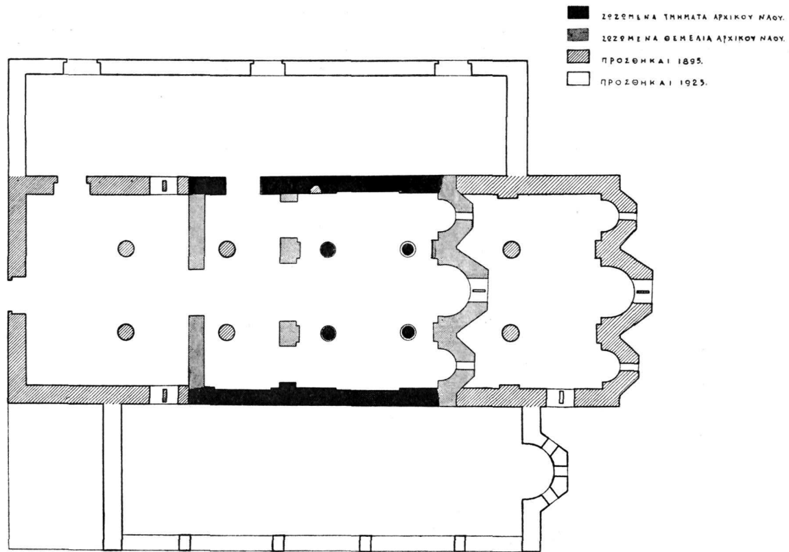
Εἰκ. 1. Ναός Ἀσωμάτων. Κάτωφιν τοῦ μνημείου πρὸ τῶν ἐργασιῶν.
