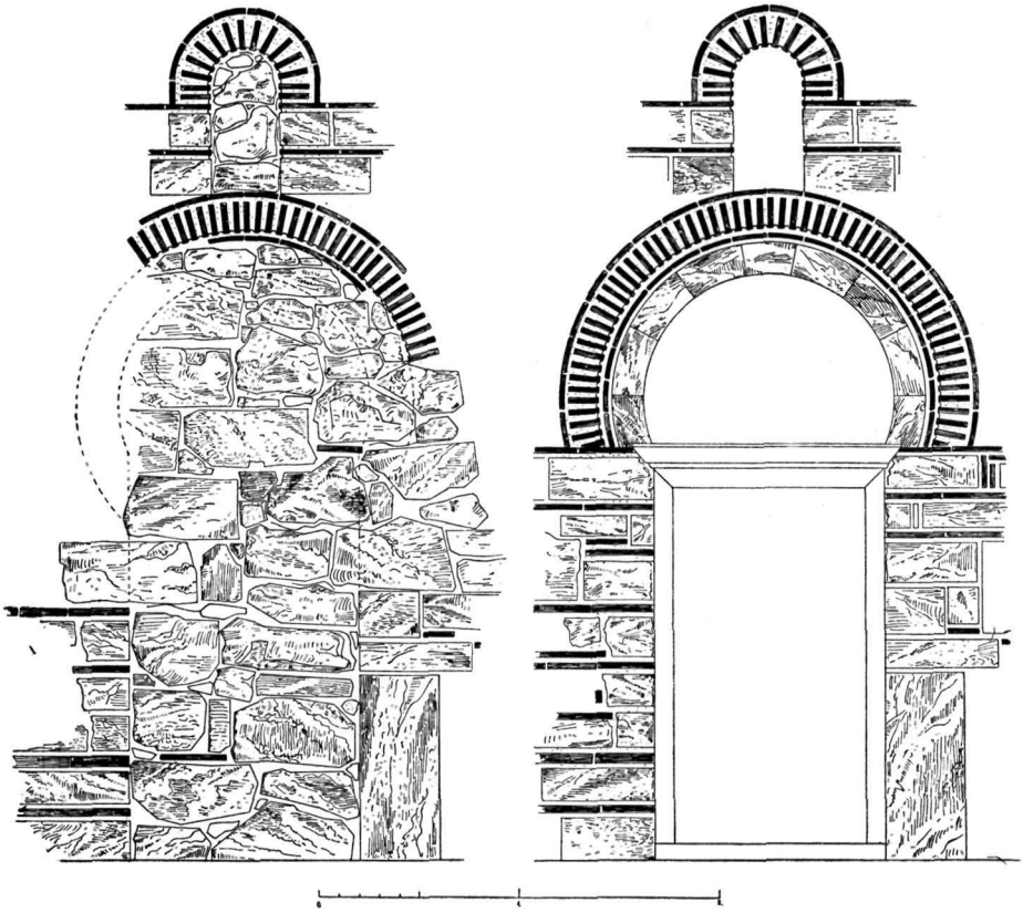
Εἰκ. 3. Θύρα με πεταλόμορφον τόξον εἰς τὴν βορείαν πλευρὰν τοῦ νάρθηκος. Μορφή, τὴν ὁποίαν εἶχε κατὰ τὴν εὐρεσίαν της, καὶ ἀποκατάστασις τοῦ ἀρχικοῦ της σχήματος.
