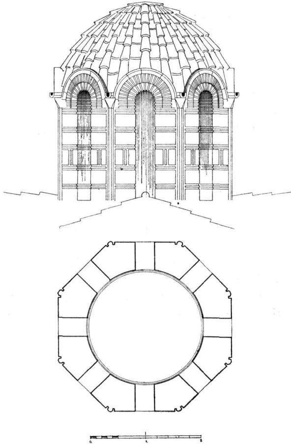
Εἰκ. 7. Ναὸς Ἁγ. Ἀσωμάτων. Τομὴ καὶ ὄψεις τοῦ τρούλλου.
