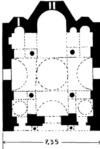
Εἰκ. 8. Ἅγιος Ἰωάννης Θεολόγος Ὑμηττοῦ. Ἄπλοῦς τετράστυλος Κωνσταντινουπόλεως.
