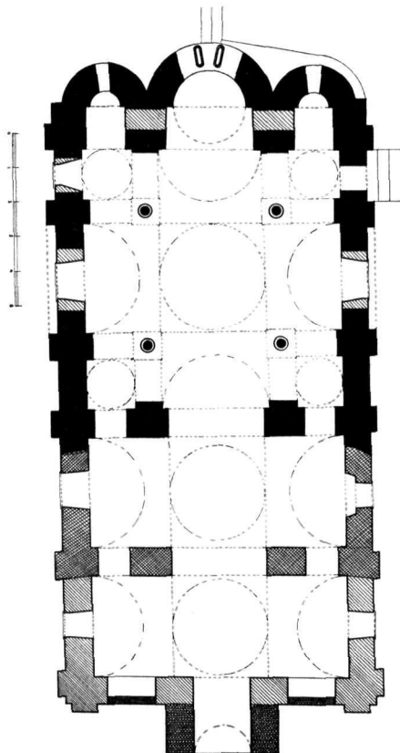
Εἰκ. 1. Κάτοψις τοῦ Καθολικοῦ τῆς Μονῆς Πετράκη.
