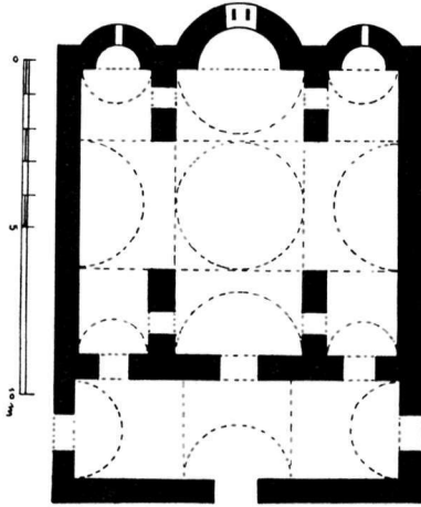
Εἰκ. 4. Παναξιώτισσα Γαυρολίμνης. Ἐπαρχιακὸς μεταβατικὸς τύπος.
