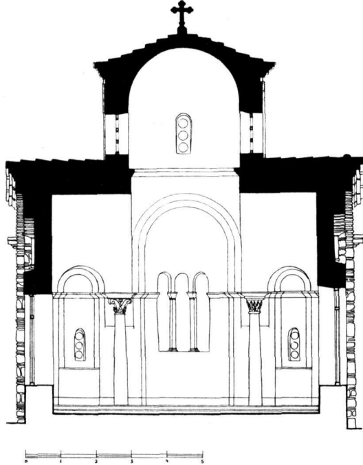
Εἰκ. 2. Τομή κατὰ πλάτος τοῦ Καθολικοῦ τῆς Μονῆς Πετράκη.
