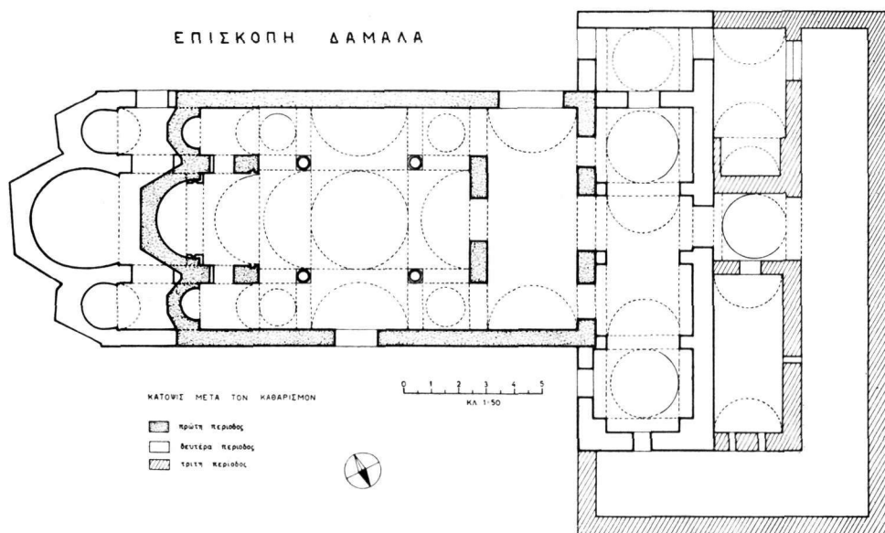
Εἰκ. 3. Κάτοψις τῆς Ἐπισκοπῆς Δαμαλᾶ μετὰ τὰς προσφάτους ἐργασίας.
