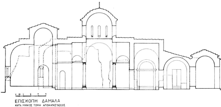
Εἰκ. 9. Κατὰ μῆκος τομὴ τῆς ἀποκαταστάσεως τοῦ ναοῦ κατὰ τὴν τελευταίαν περίοδον.
