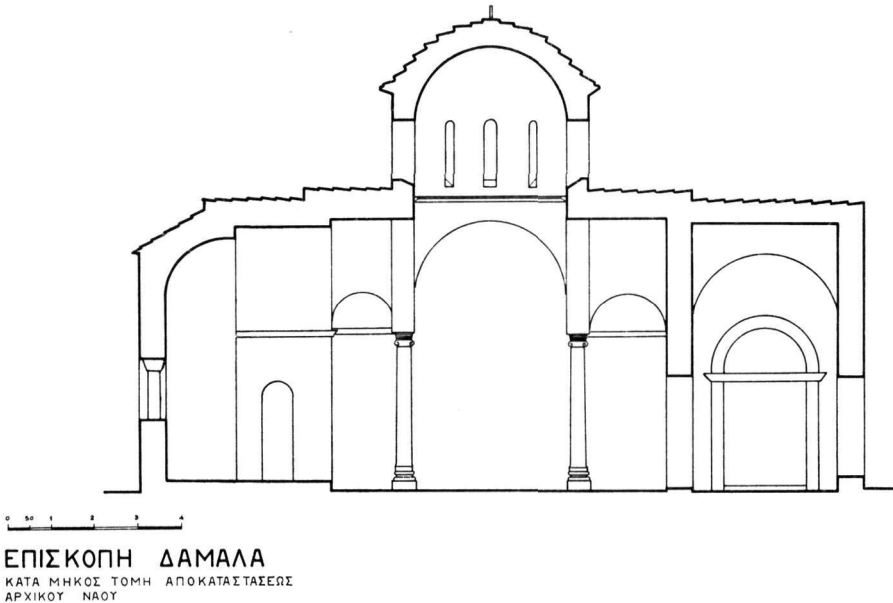
Εἰκ. 6. Κατὰ μῆκος τομὴ ἀποκαταστάσεως ἀρχικοῦ ναοῦ.
