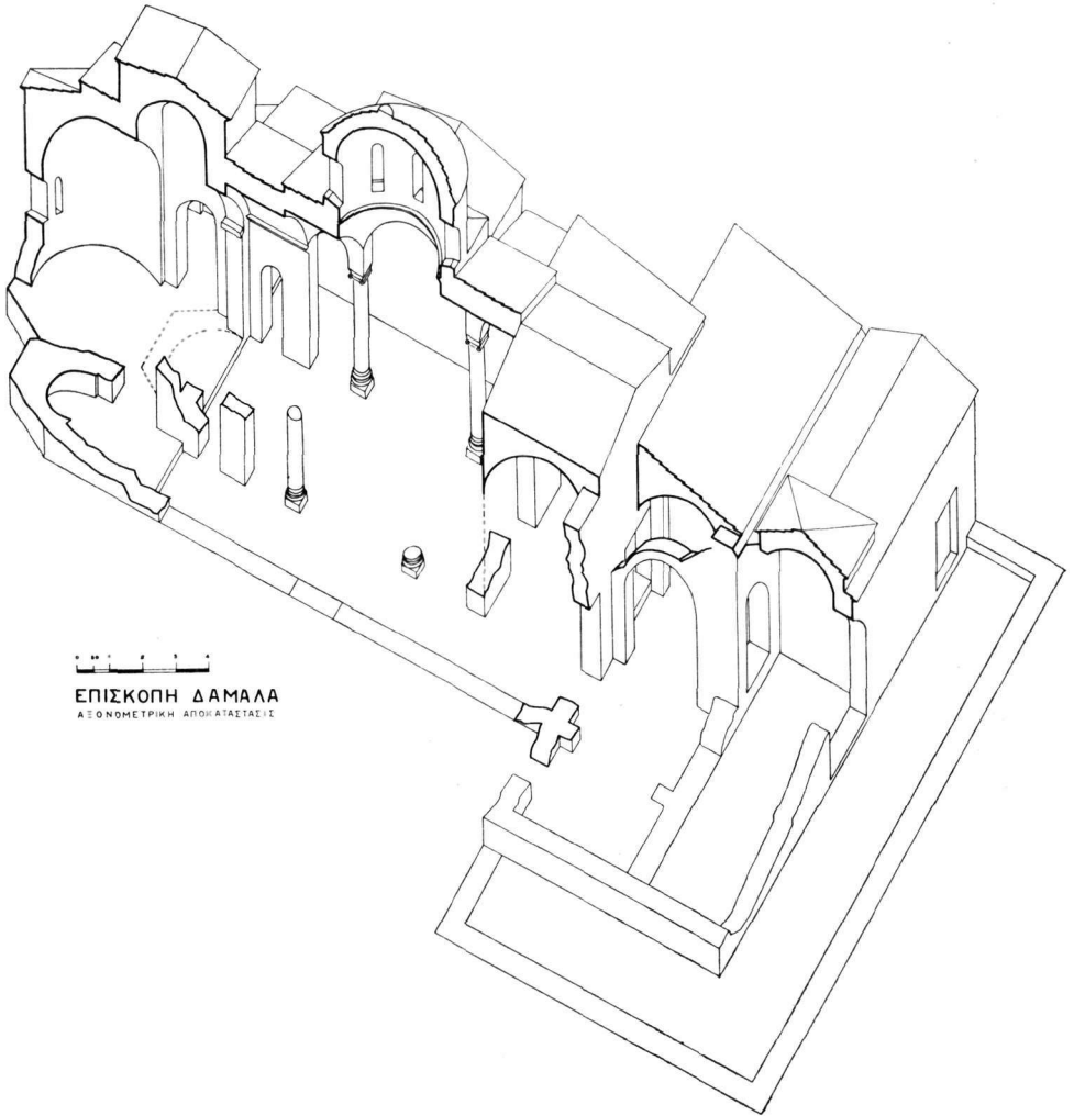
Εἰκ. 10. Ἀξονομετρικὴ ἀποκατάστασις τοῦ ναοῦ κατὰ τὴν τελευταίαν περίοδον.
