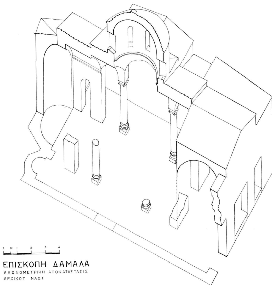
Εἰκ. 7. Ἀξονομετρικὴ ἀποκατάστασις ἀρχικοῦ ναοῦ.
