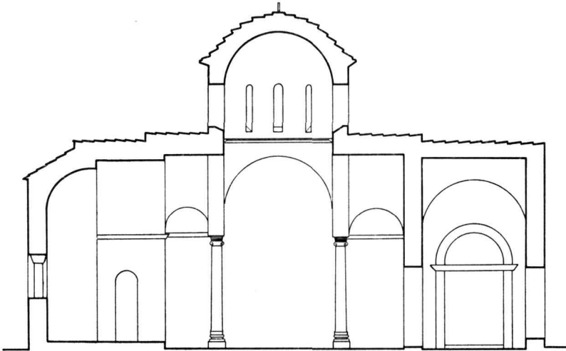
ΕΠΙΣΚΟΠΗ ΔΑΜΑΛΑ ΚΑΤΑ ΜΗΚΟΣ ΤΟΜΗ ΑΠΟΚΑΤΑΣΤΑΣΕΩΣ ΑΡΧΙΚΟΥ ΝΑΟΥ
