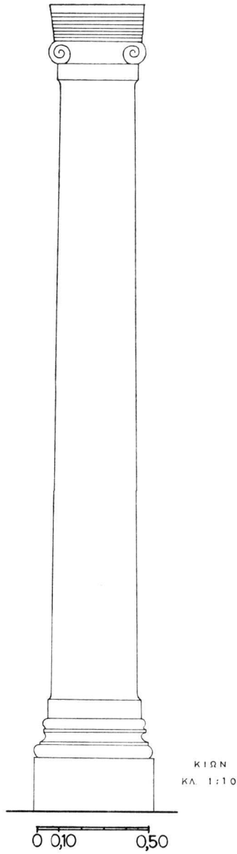
Εἰκ. 5. Μαρμάρινος κίων τοῦ ἀρχικοῦ ναοῦ τῆς Ἐπισκοπῆς τοῦ Δαμαλά.
