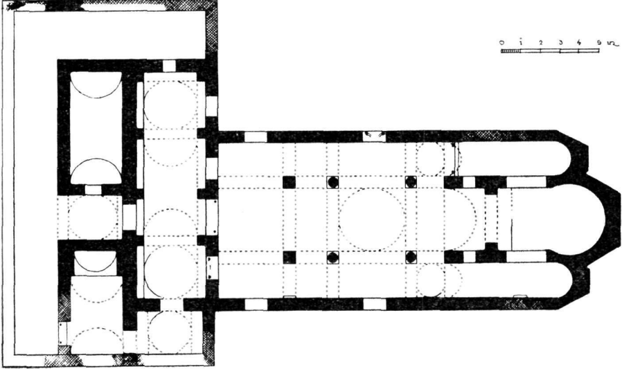
Εἰκ. 2. Κάτοπις τῆς Ἐπισκοπῆς Δαμαλᾶ κατὰ G. Welter.
