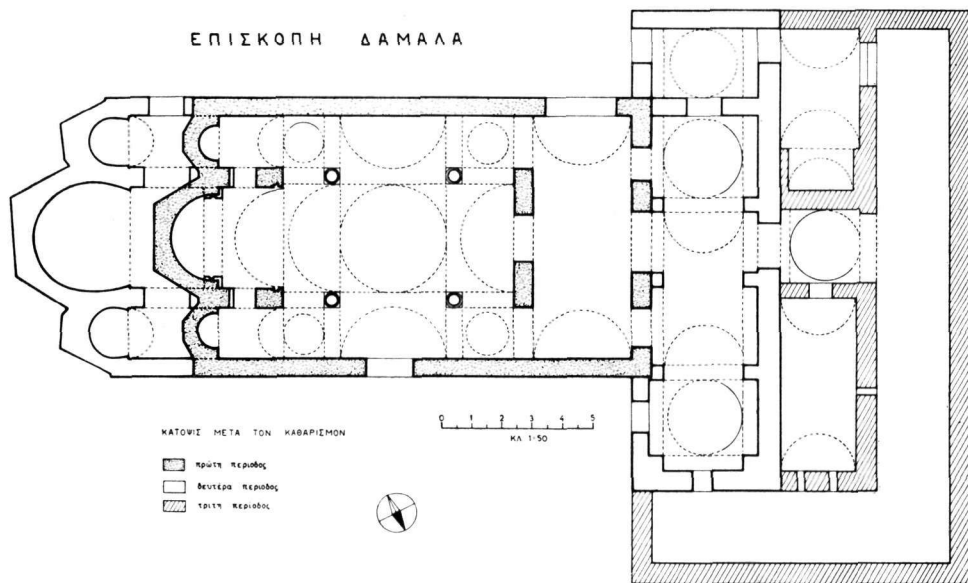
Εἰκ. 3. Κάτωσις τῆς Ἐπισκοπῆς Δαμαλᾶ μετὰ τὰς προσφάτους ἐργασίας.
