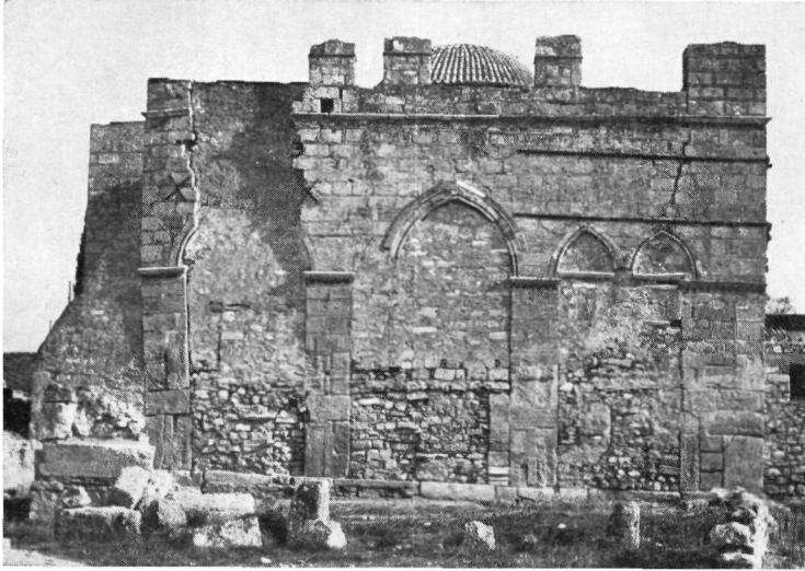
1. Δυτική ὄψις τοῦ ἔξωνάρθηκος πρὸ τῆς ἀναστηλώσεως.
