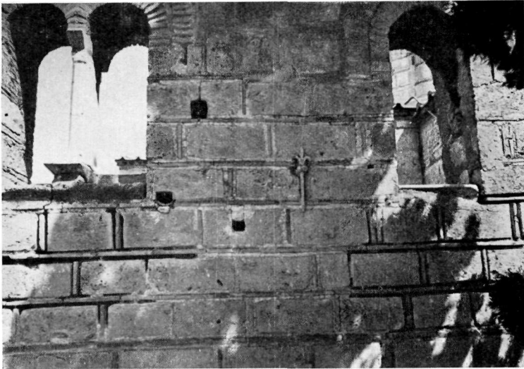
3. Πλινθοπερίβλητον σύστημα τοιχοποιΐας ἄνωθεν τῶν τριλόβων παραθύρων τῆς νοτίας πλευρᾶς μετὰ πάχος πλίνθου 2,5 ἐκ.
