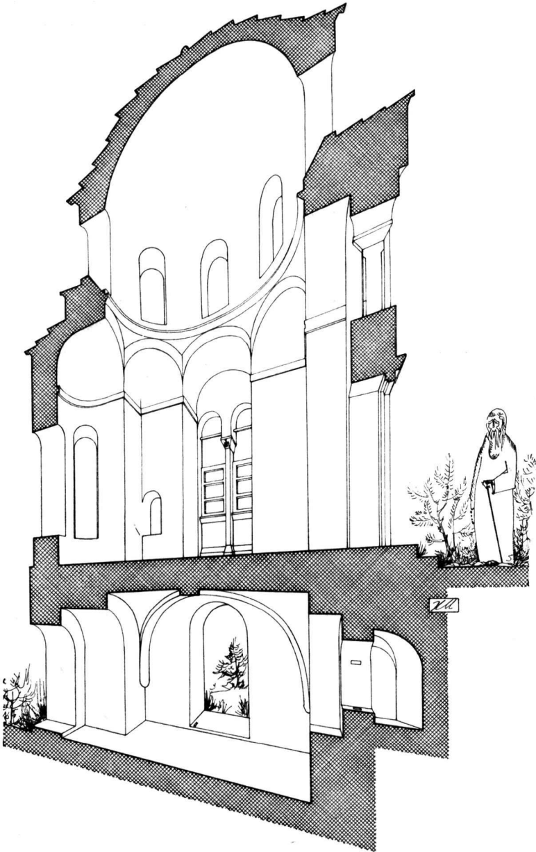
Εἰκ. 9. Ναῖσκος Ὁσίου Λουκᾶ. Ἀναπαράστασις τῆς ἀρχικῆς μορφῆς τοῦ μνημείου. Προοπτικὴ τομὴ.
