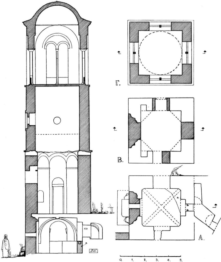
Εἰκ. 1. Κωδωνοστάσιον Ὁσίου Λουκά. Ὑπάρχουσα κατάστασις. Τομὴ κατὰ μῆκος καὶ κατόψεις πρώτου, δευτέρου καὶ τετάρτου ὀρόφου.
