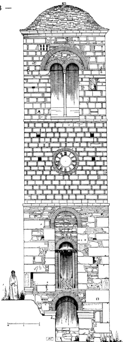
Εἰκ. 2. Κωδωνοστάσιον Ὀσίου Λουκά. Ὑπάρχουσα κατάστασις. Νοτιὰ ὄψις.
