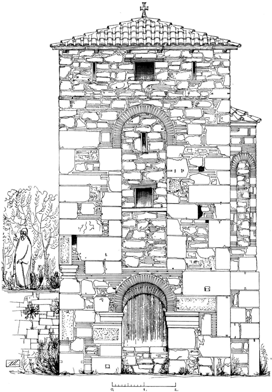
Εικ. 7. Ναΐσκος Ὁσίου Λουκά. Ἀναπαράστασις τοῦ μνημείου κατὰ τὸν 18 ο αἰῶνα. Νοτία ὄψις.
