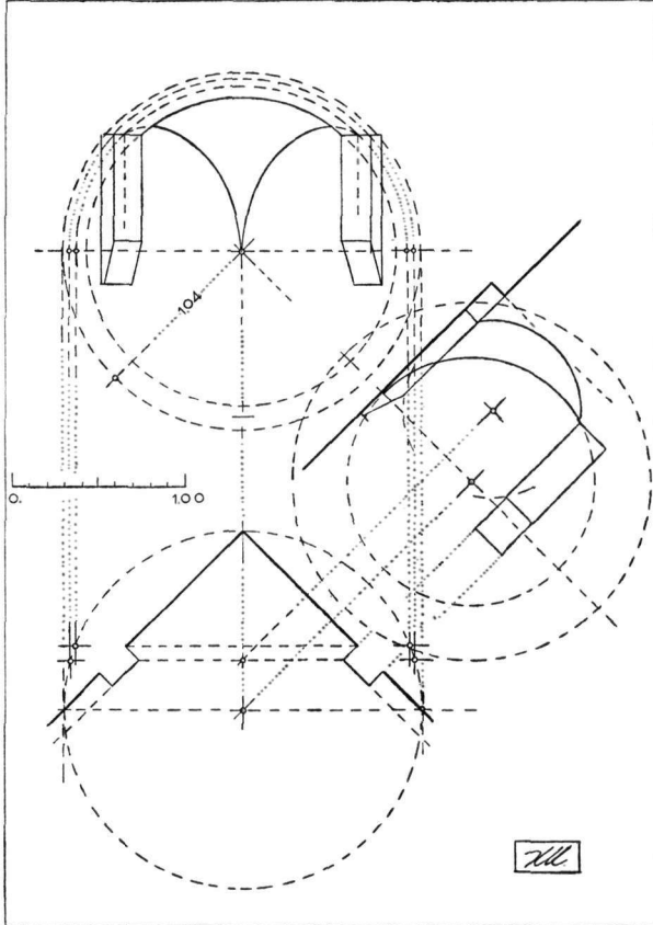
Εἰκ. 11. Ἅγιος Ἰωάννης Κέρου. Γεωμετρικὴ ἐρμηνεῖα τῆς κατασκευῆς τῶν ἡμιχωνίων. Κάτοψις, ὄψις πλαγία καὶ ὄψις κατὰ τὴν διαγώνιον.
