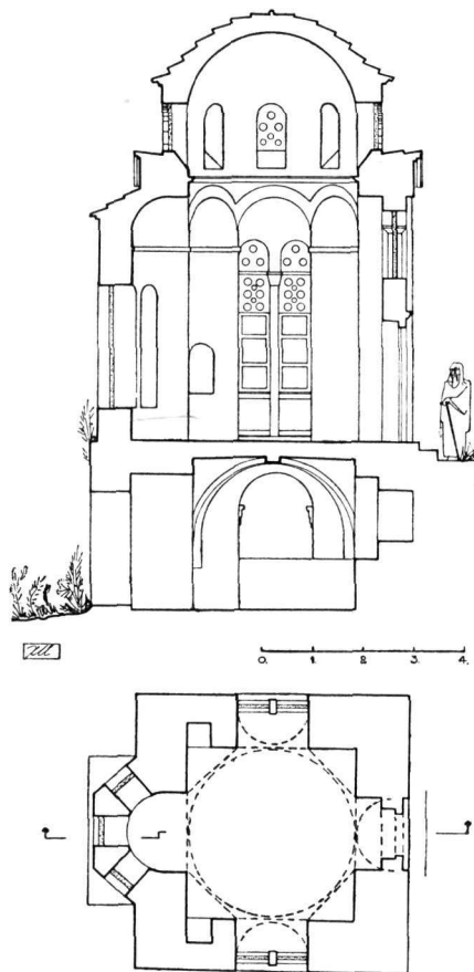
Εἰκ. 4. Ναῖσκος Ὁσίου Λουκά. Ἀναπαράστασις τῆς ἀρχικῆς μορφῆς τοῦ μνημείου. Κάτοψις τοῦ ὀρόφου καὶ τομὴ κατὰ μήκος.
