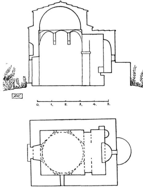
Εἰκ. 10. Ἅγιος Ἰωάννης Κέρους. Κάτοψις καὶ τομὴ κατὰ μῆκος.
