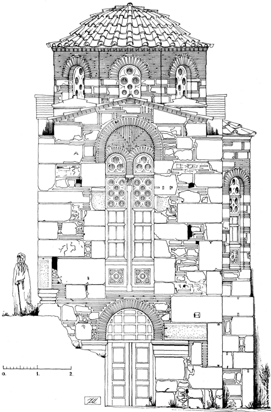
Εἰκ. 5. Ναῖσκος Ὁσίου Λουκᾶ. Ἀναπαράστασις τῆς ἀρχικῆς μορφῆς τοῦ μνημείου. Νοτία ὄψις.
