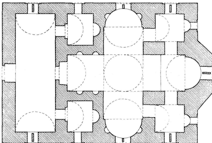
Εικ. 3. "Άγιος Νικόλαος Αΰλιδος. Κάτοψις και κατά μήκος τομή. "Αναπαράστασις.
