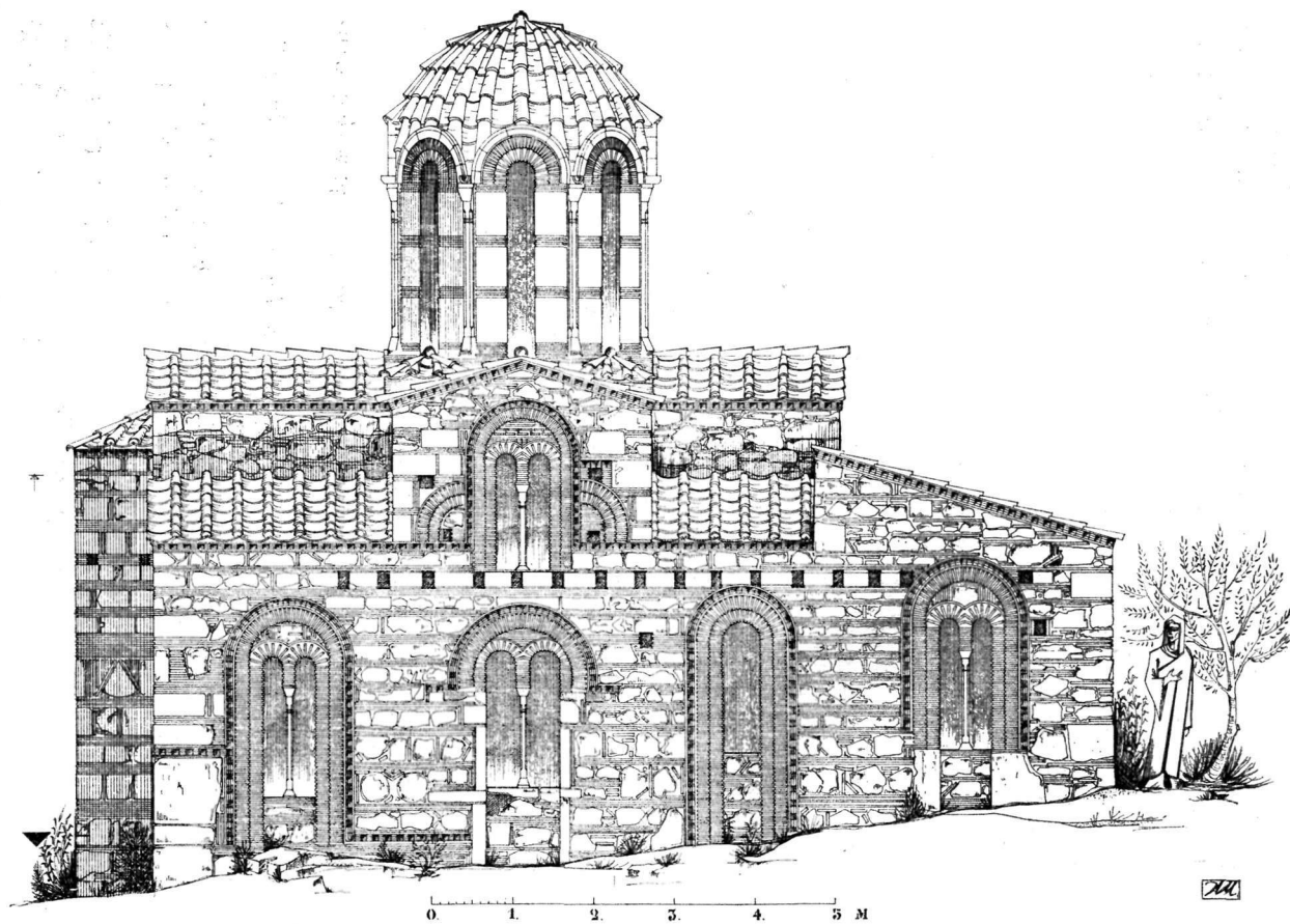
Εικ. 5. "Άγιος Νικόλαος Αύλιδος, Βορειαί ὄψεις. Ἐναπαράστασις.
