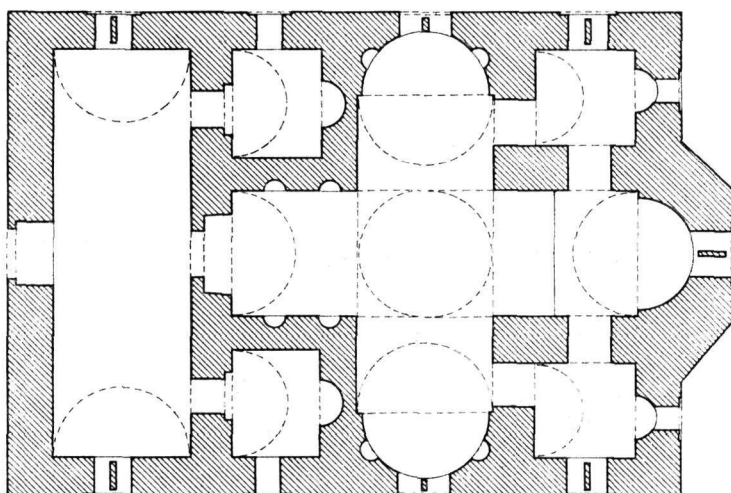
Εικ. 3. "Άγιος Νικόλαος Αΰλιδος. Κάτοψις και κατὰ μήκος τομή. "Αναπαράστασις.
