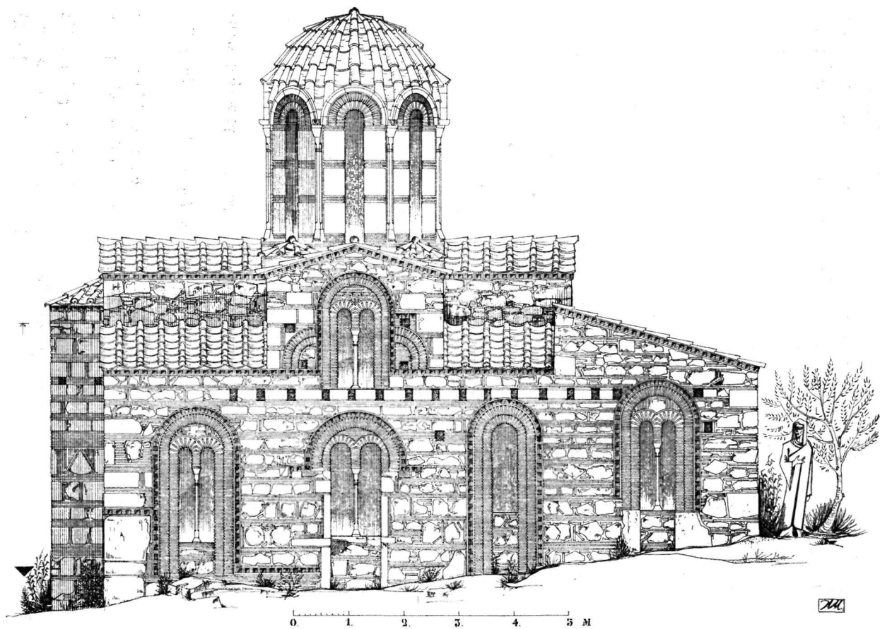
Εικ. 5. "Άγιος Νικόλαος Αΰλιδος, Βορεια ὄψις. Ἐναπαράστασις.
