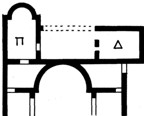
Εἰκ. 22. Κάτοψις τοῦ ἱεροῦ τῆς βασιλικῆς Ἁγλαδεργῆς Λέσβου.
