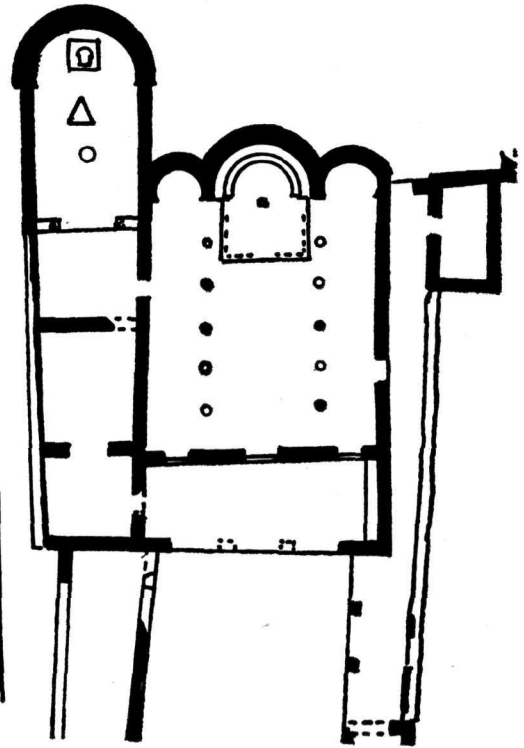
Εἰκ. 24. Κάτοψις τῆς βασιλικῆς τοῦ Κιριπάτ-αλ-Καράκ.
