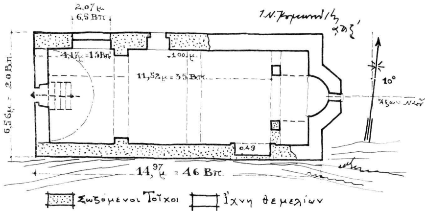
Σχέδ. 2. Ἅγιοι Ἀπόστολοι. Κάτοψις μετὰ συμπληρώσεων.
