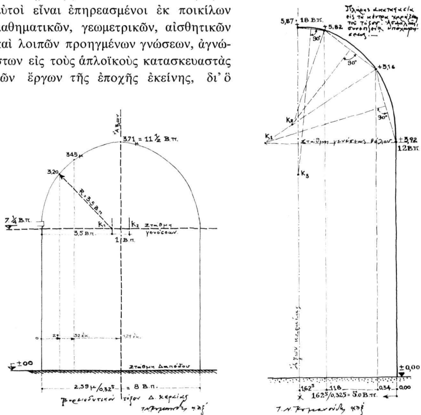
Σχέδ. 9, 10. Κοίμησις. Λεπτομέρεια χαράξεως τόξων.
