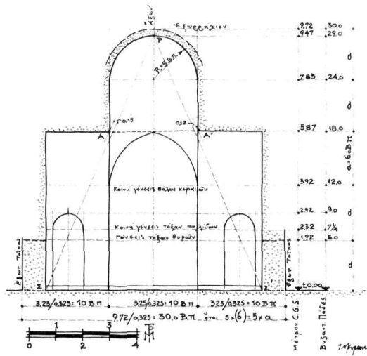
Σχέδ. 8. Κοίμησις. Ἐγκαρσία τομή. Διακρίνεται ὁ τεκτονικὸς κἀνναβος καὶ τὸ μὴ ἐγγράμμιον ἰσοσκελὲς τρίγωνον.
