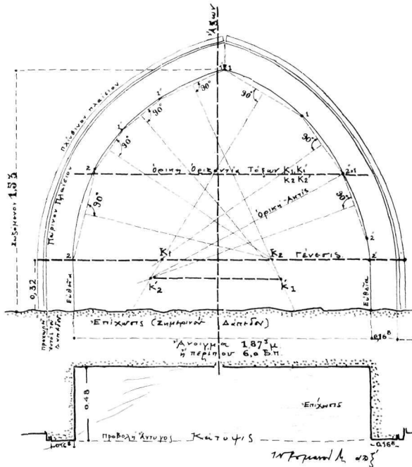
Σχέδ. 3. Ἁγιοὶ Ἀπόστολοι. Γεωμετρικὴ ἀνάλυσις τόξου κόγχης Ν. τοίχου.
