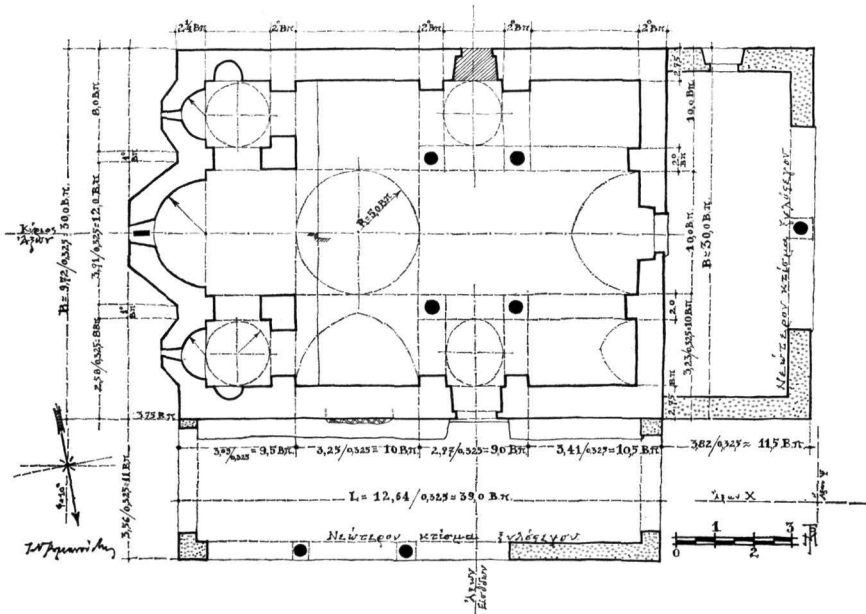
Σχέδ. 6. Κοίμησις. Κάτωρις, ένθα έμφανίζεται ό τεκτονικός κάναβος.
