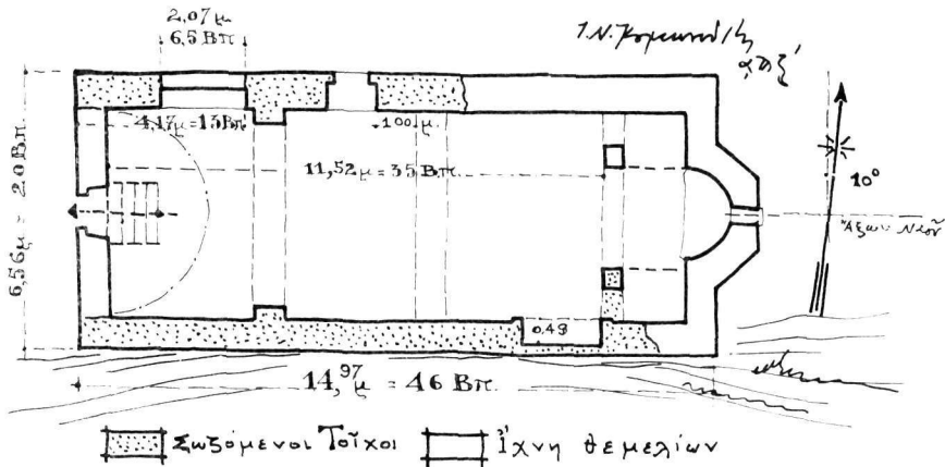
Σχέδ. 2. ᾽Αγιοὶ Ἀπόστολοι. Κάτοψις μετὰ συμπληρώσεων.
