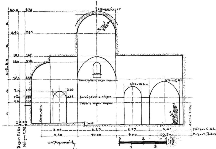
Σχέδ. 7. Κοίμησις. Κατὰ μῆκος τομῇ. Διακρίνεται ὁ τεκτονικὸς κἀνναβος.
