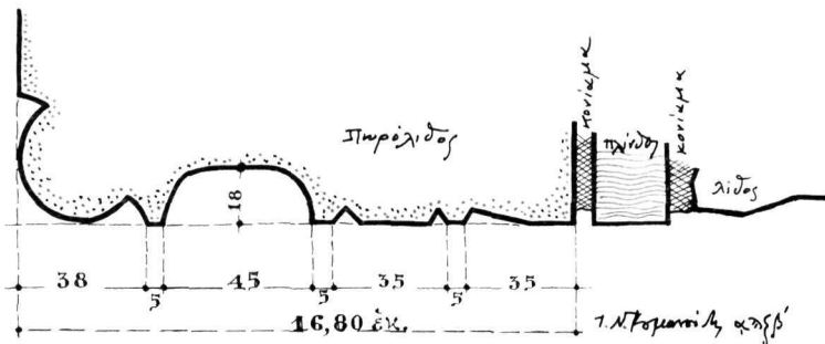
Σχῆδ. 4. Ἅγιοι Ἀπόστολοι. Λεπτομέρεια πυρίνου κυματίου.
