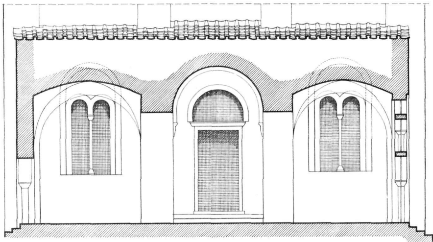
Εἰκ. 2. Κατὰ μῆκος τομή τοῦ ἐξωνάρθηκα (ἀποκατάσταση).
