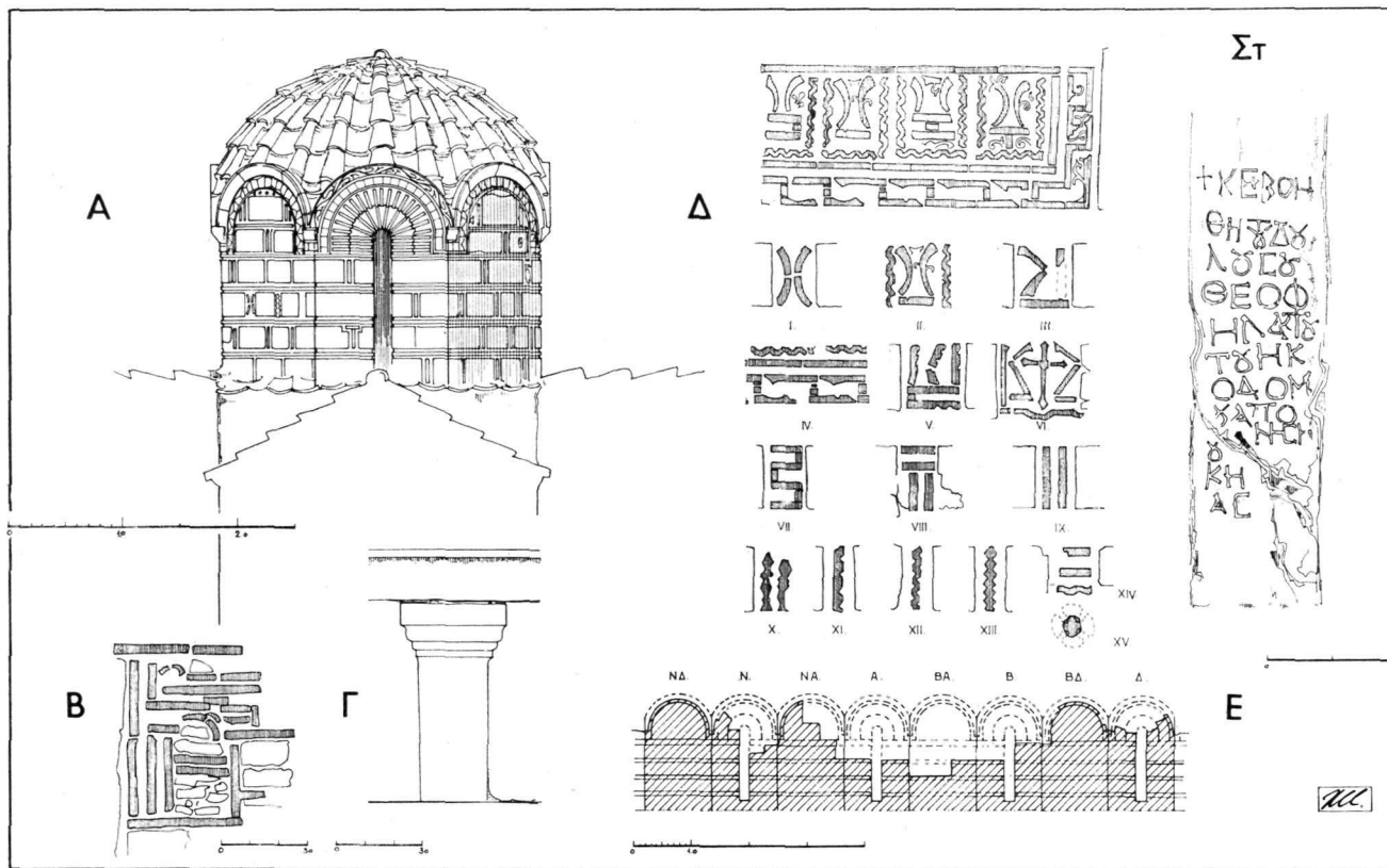
Εικ. 6. *Άγιος Ιωάννης Λιγουριού. Α) Αναπαράσταση του τρούλλου του ναού Β) Κόσμημα από τουβλα στην βόρεια όψη. Γ) Η Άγία Τράπεζα. Δ) Τά κεραμικά κοσμήματα του ναού. Ε) Ανάπτυγμα του τυμπάνου του τρούλλου (τά σκιαζόμενα μέρη παραμένουν τὰ ἀρχικά). Στ) Έπιγραφή στην παραστάδα της βόρειας εισόδου.
