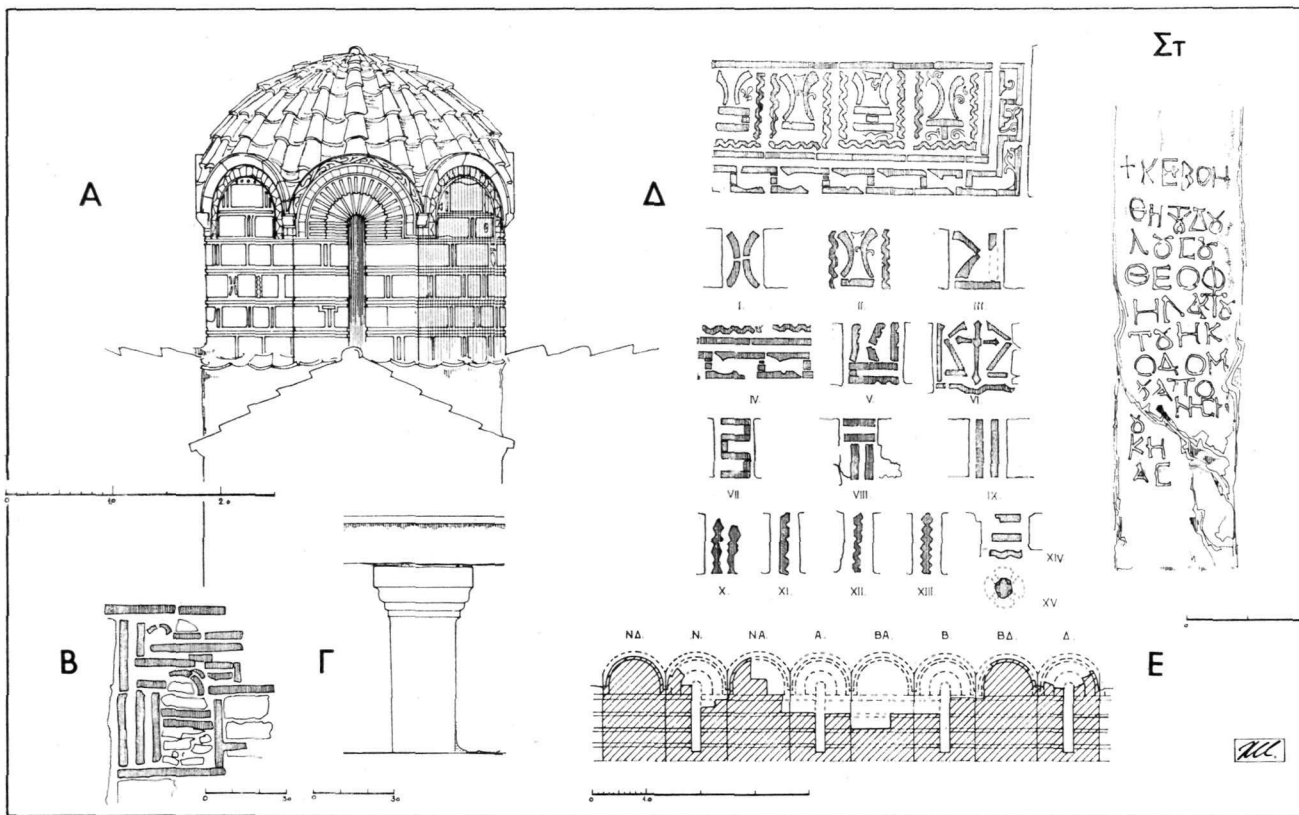
Εικ. 6. *Άγιος Ιωάννης Λιγουριοῦ. Α) Ἀναπαράσταση τοῦ τροῦλλου τοῦ ναοῦ Β) Κόσμημα ἀπὸ τοῦβλα στὴν βόρεια ὄψη. Γ) Ἡ Ἁγία Τράπεζα. Δ) Τὰ κεραμικὰ κοσμήματα τοῦ ναοῦ. Ε) Ἀνάπτυγμα τοῦ τυμπάνου τοῦ τροῦλλου (τὰ σκιαζόμενα μέρη παραμένουν τὰ ἀρχικά). Στ) Ἐπιγραφή στὴν παραστάδα τῆς βόρειας εἰσόδου.
