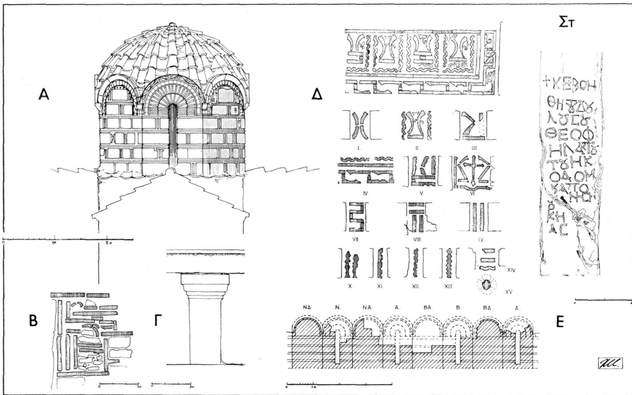
Εικ. 6. *Άγιος Ίωάννης Λιγουριοῦ. Α) Ἀναπαράσταση τοῦ τροῦλλου τοῦ ναοῦ Β) Κόσμημα ἀπὸ τοῦβλα στὴν βόρεια ὄψη. Γ) Ἡ Ἁγία Τράπεζα. Δ) Τὰ κεραμικὰ κοσμήματα τοῦ ναοῦ. Ε) Ἀνάπτυγμα τοῦ τυμπάνου τοῦ τροῦλλου (τὰ σκιαζόμενα μέρη παραμένουν τὰ ἀρχικά). Στ) Ἐπιγραφή στὴν παραστάδα τῆς βόρειας εἰσόδου.
