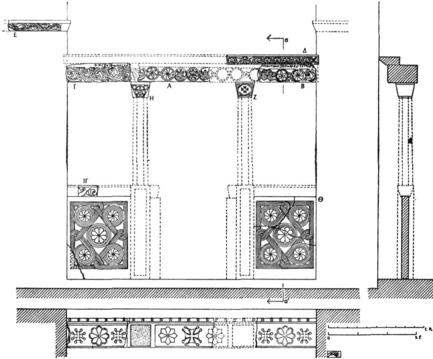
Εικ. 1. Χίος. Παναγία Κρίνα. Τò μαρμαρίνο τέμπλο σέ αναπαράσταση. Όψη, άνοψη και τομή.
