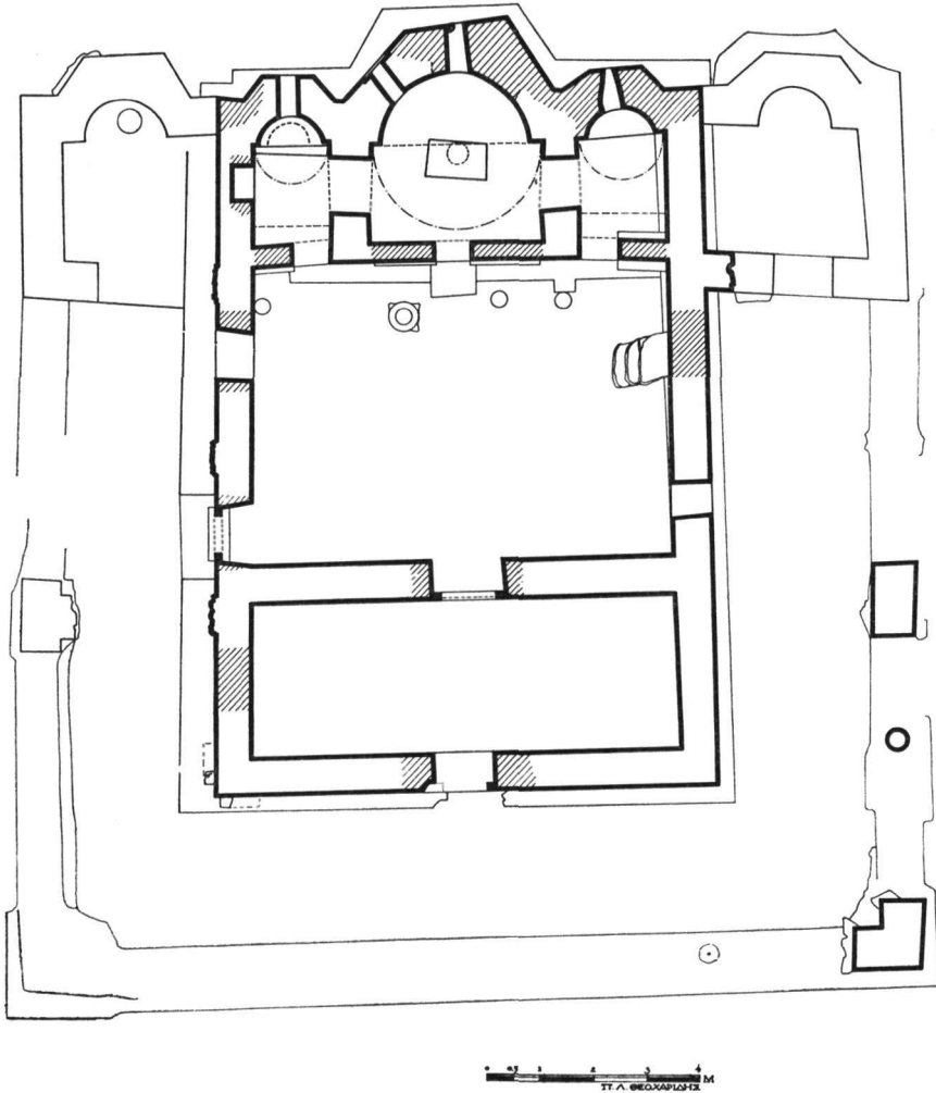
Εἰκ. 1. Μοναστηράκι Βονίτισης. Ναὸς Παντοκράτορος. Κάτοψη.
