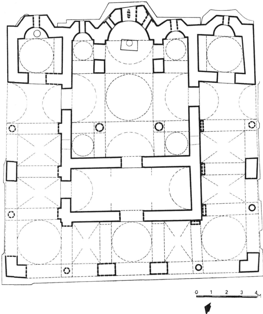
Εἰκ. 2. Μοναστηράκι Βονίτσης. Ναὸς Παντοκράτορος. Ἀναπαράσταση τῆς κατόψεως.
