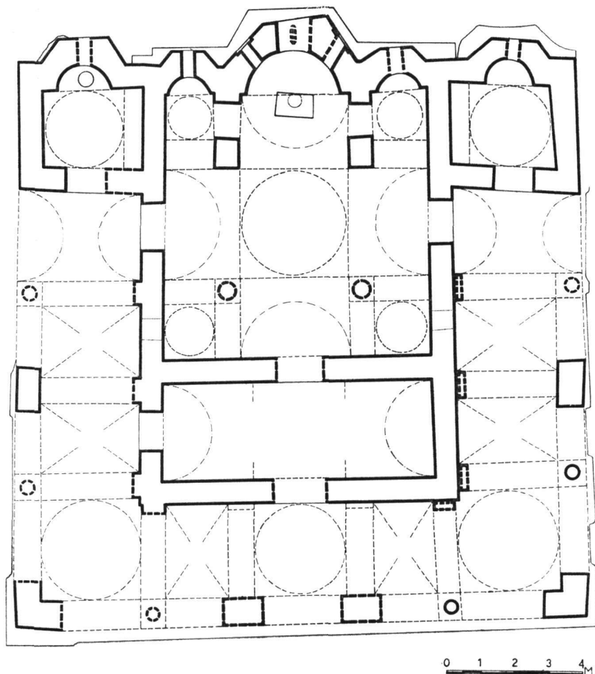
Εἰκ. 2. Μοναστηράκι Βονίτσης. Ναὸς Παντοκράτορος. Ἀναπαράσταση τῆς κατόψεως.
