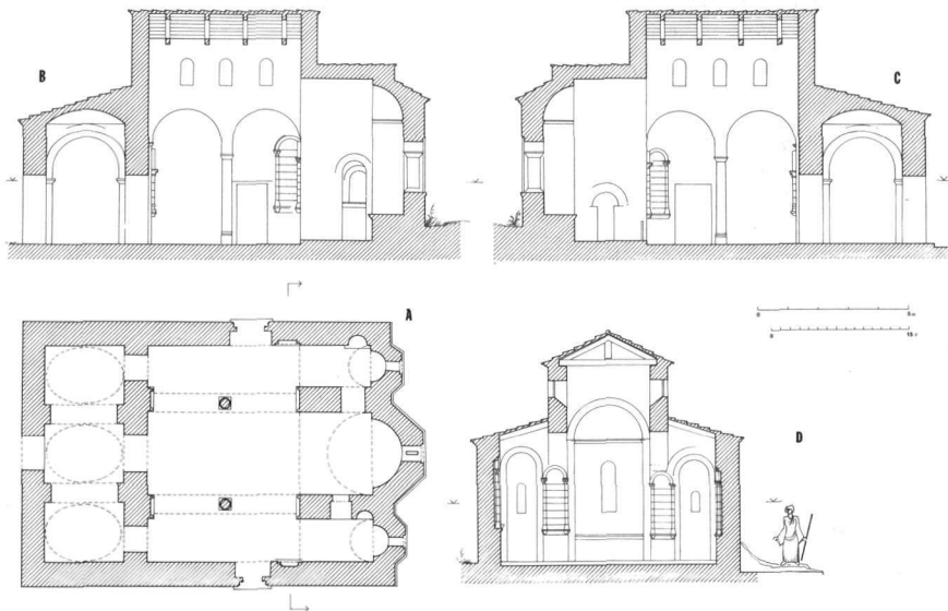
Εἰκ. 16. Θεοτόκος Ἄνηλιου. Κάτοψη, δύο τομές κατά τό μήκος καί τομή κατά τό πλάτος τοῦ ναοῦ, σέ ἀναπαράσταση.
