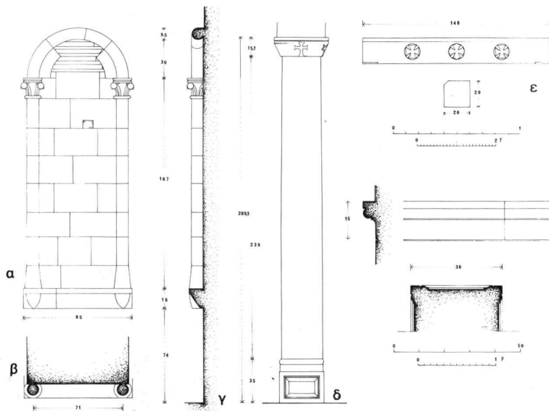
Εικ. 4. Θεοτόκος Ἀνηλίου. Λεπτομέρειες σέ ἀναπαράσταση: α. Προσκυνητᾶρι πεσοῦ τοῦ ἱεροῦ σέ κάτοψη καί τομή. β. Ἐνας ἀπό τούς κίονες. γ. Τό ὑπέρθυρο σέ ὄψη καί τομή. δ. Ὁ πῶρινος κοσμητῆς τοῦ ἱεροῦ σέ ὄψη καί τομή. ε. Τό βάθρο τοῦ κίονος σέ τομή.
