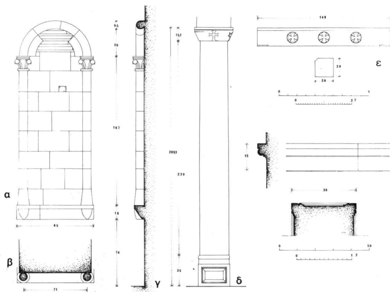
Εικ. 4. Θεοτόκος Ἀνηλίου. Λεπτομέρειες σέ ἀναπαράσταση: α. Προσκυνητάρι πεσσού τοῦ ἱεροῦ σέ κάτοψη καί τομή. β. Ἐνας ἀπό τούς κίονες. γ. Τό ὑπέρθυρο σέ ὄψη καί τομή. δ. Ὁ πῶρινος κοσμήτης τοῦ ἱεροῦ σέ ὄψη καί τομή. ε. Τό βάθρο τοῦ κίονος σέ τομή.
