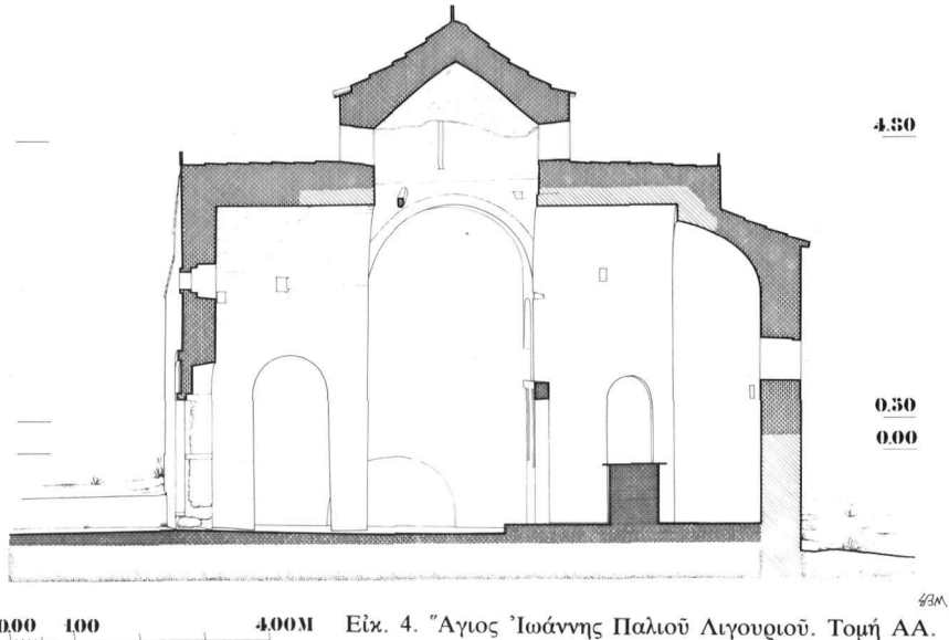
0.00 100 4.00M Εικ. 4. Ἅγιος Ἰωάννης Παλιού Λιγουριού. Τομή ΑΑ.
