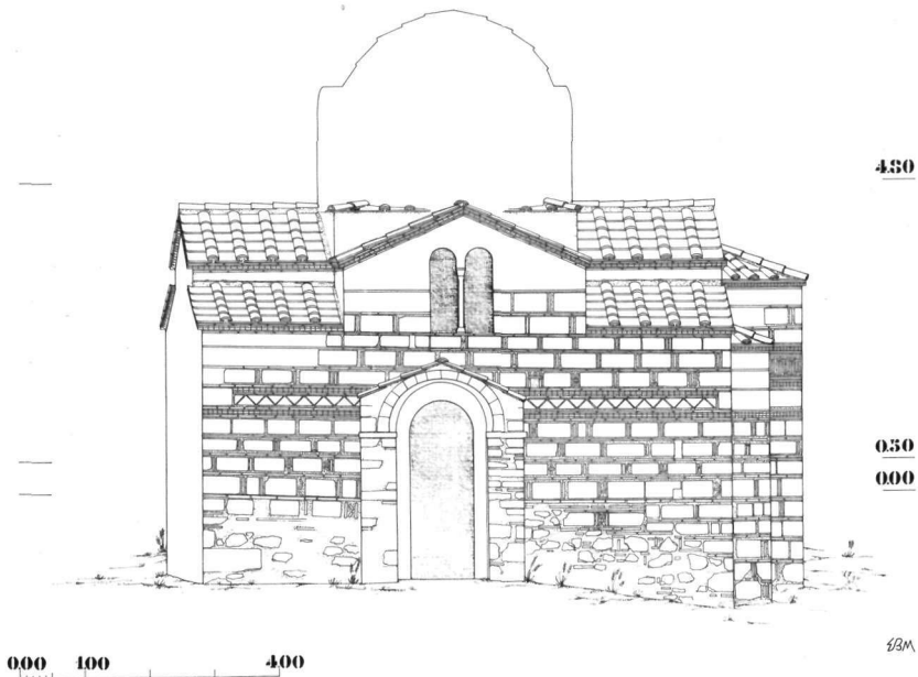
Είχ. 14. Ἅγιος Ἰωάννης Παλιῶ Λιγουριῶ. Νότια ὄψη. Ἀναπαράσταση.
