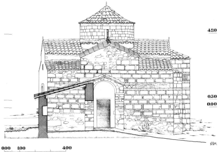
Είχ. 13. Άγιος Ίωάννης Παλιού Λιγουριού. Νότια όψη. Έγάρχουσα κατάσταση.
