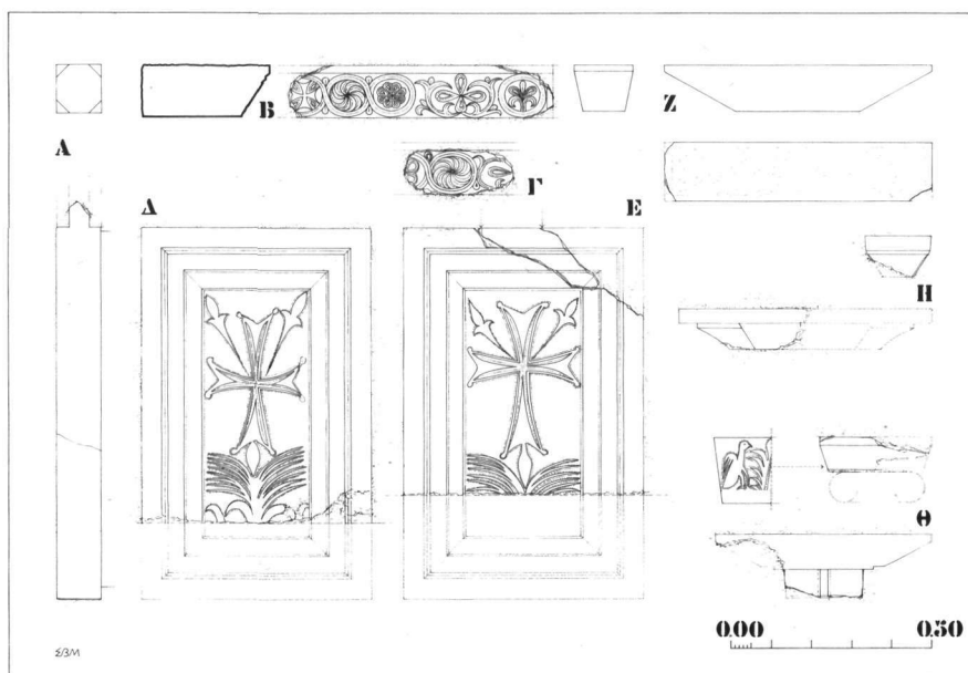
Εικ. 7. "Άγιος Ἰωάννης Παλιού Λιγουριού. Μαρμάρινα ἀρχιτεκτονικά μέλη ἐνσωματωμένα στό μνημεῖο. Α. Πεσόσκος τέμπλου. Β. Θραύσμα ἐπιστυλίου τέμπλου. Γ. Θραύσμα ἐπιστυλίου τέμπλου. Δ καί Ε. Θωράκια. Ζ καί Η. Ἐπιθήματα ἀμφικιονίσκων. Θ. Ἐπίθημα συμφυές μέ ἰωνικό κιονοκρανο.
