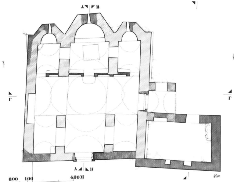
Είκ. 3. Ἅγιος Ἰωάννης Παλίου Λιγουρίου. Κάτοψη.
