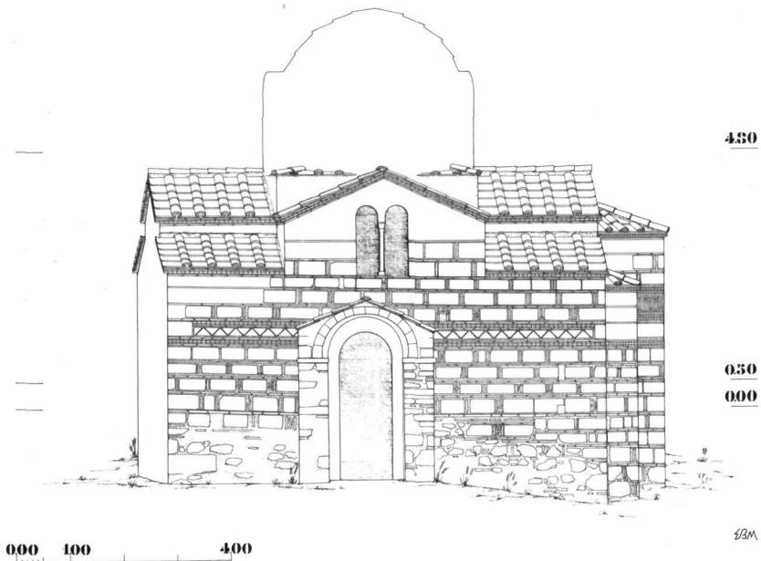
Είχ. 14. Άγιος Ίωάννης Παλιού Λιγουριού. Νότια όψη. 'Αναπαράσταση.
