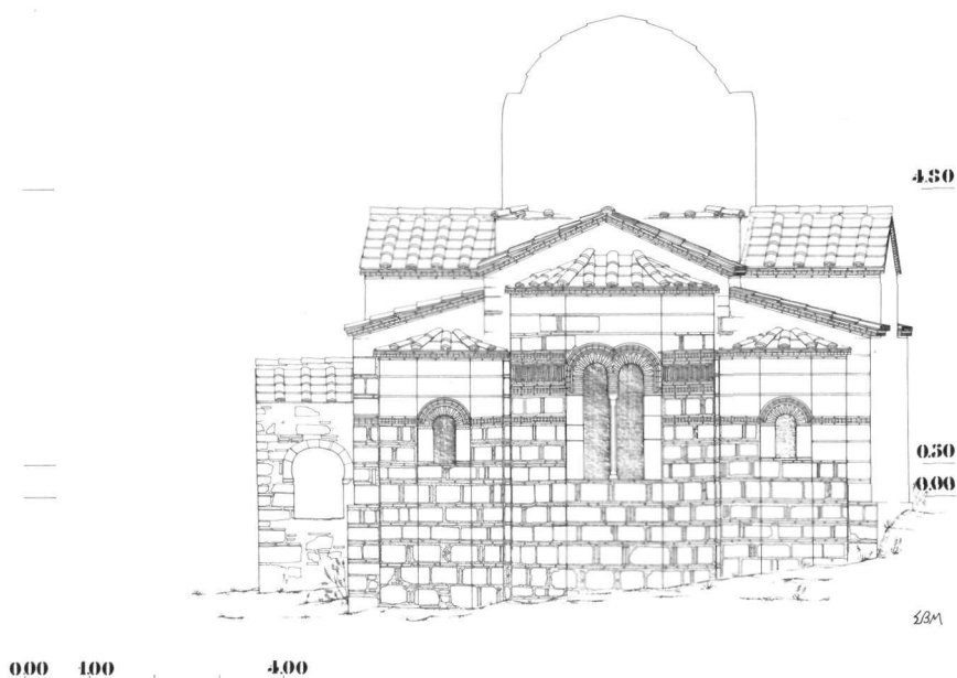
Εικ. 12. Ἅγιος Ἰωάννης Παλιῶ Λιγουριῶ. Ἀνατολική ὄψη. Ἀναπαράσταση.
