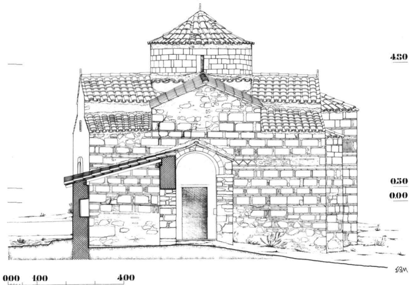
Είχ. 13. Άγιος Ίωάννης Παλιού Λιγουριού. Νότια όψη. 'Υπάρχουσα κατάσταση.
