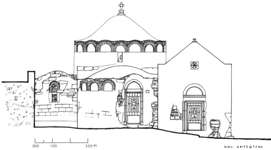
Είκ. 1. Ἐπισκοπή Ἱεράπετρας. Ἅγιος Γεώργιος-Ἅγιος Χαράλαμπος. Δυτική ὄψη. Ἀριστερά τὸ βόρειο καὶ κεντρικὸ διαμέρισμα τῆς ἀρχικῆς φάσης, δεξιὰ τὸ νεότερο κτίσις τοῦ Ἁγίου Χαράλαμπος.
