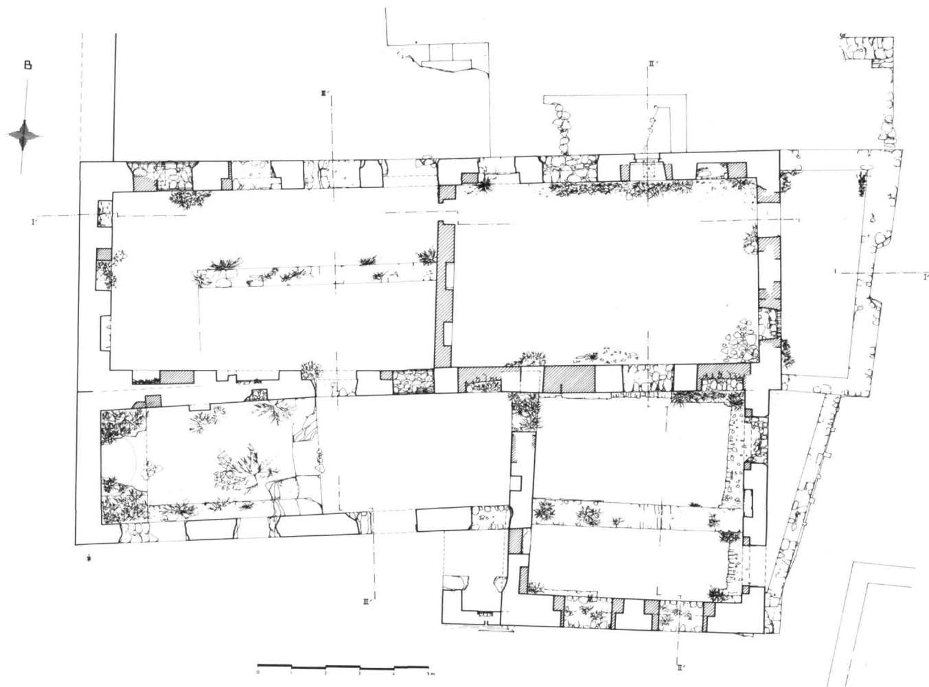
Εἰκ. 16. Σπίτι τοῦ Λάσκαρη. Τρίτη στάθμη. Κάτοψη.
