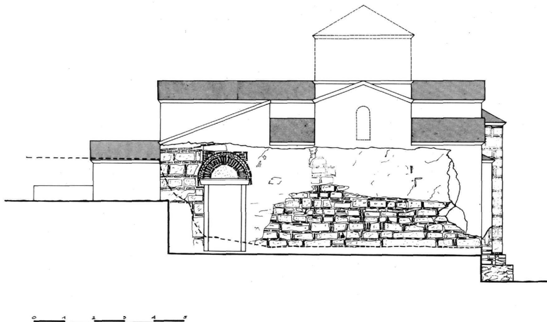
Εικ. 24. Αποκατάσταση της νότιας όψης.
