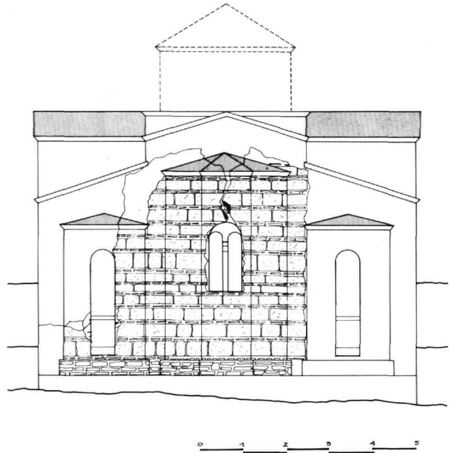
Εικ. 23. Αποκατάσταση της ανατολικής όψης.
