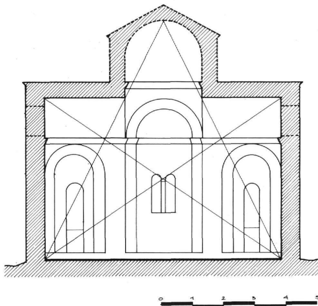
Εικ. 20. Αποκατάσταση της κατά πλάτος τομής του βυζαντινού ναού.
