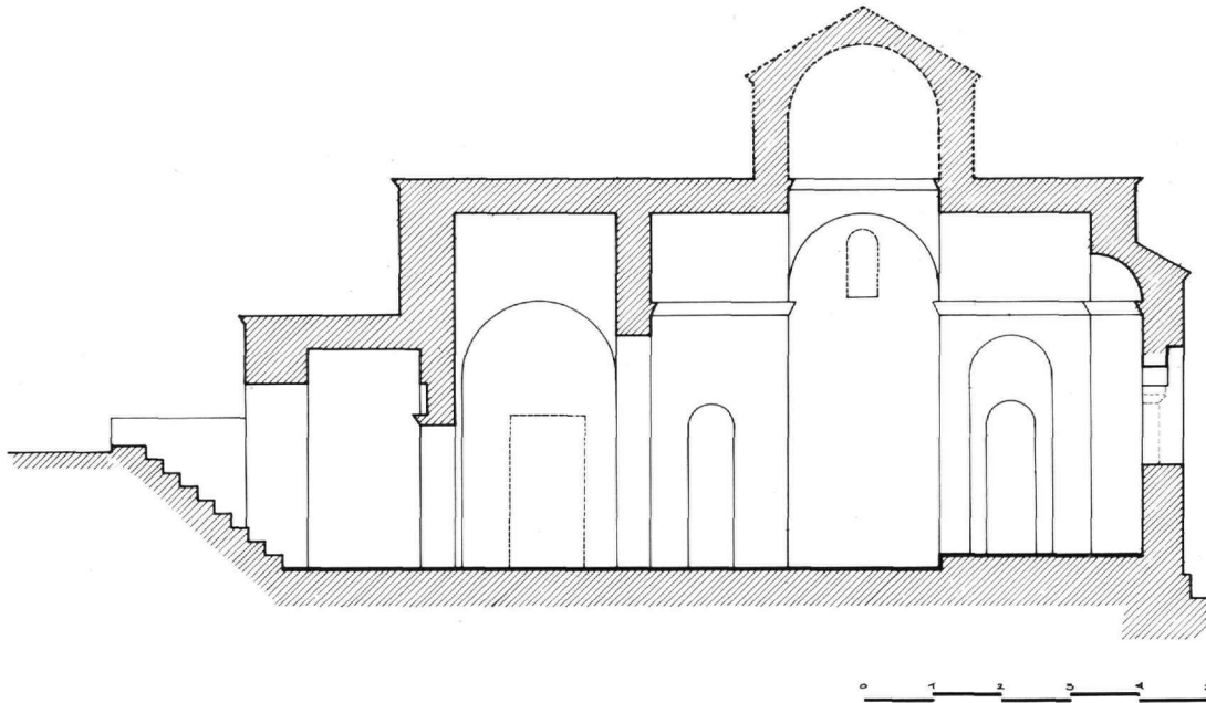
Εικ. 21. Αποκατάσταση της κατά μήκος τομής της βυζαντινής φάσης.
