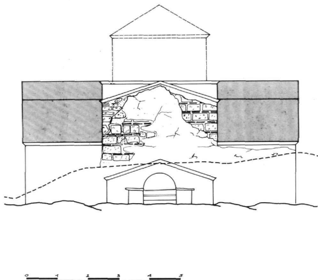
Εικ. 25. Αποκατάσταση της δυτικής όψης.
