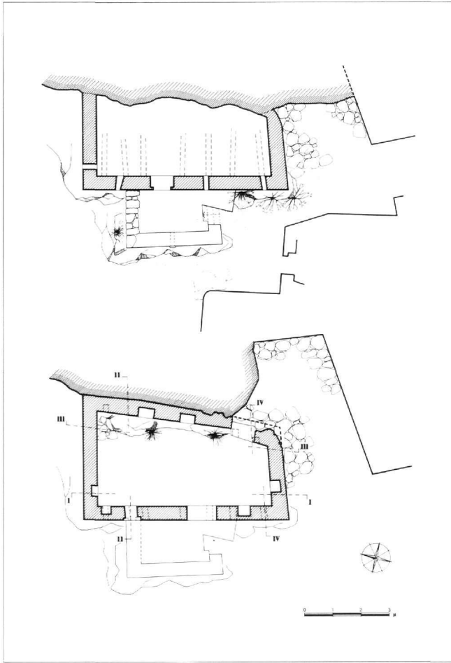
Εικ. 10. Κτίριο 8. Κάτοψη καταγίου και αναγίου.
