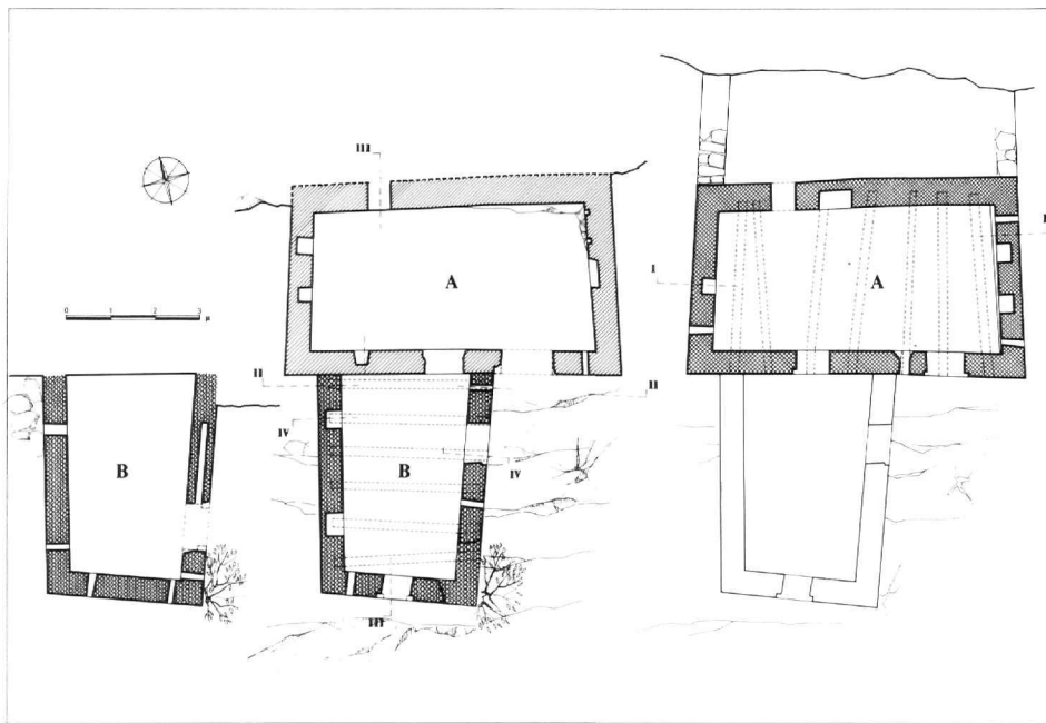
Εικ. 13. Κτίριο 2. Κάτοψη κατωγίου χώρου B, ανωγίου χώρου B και κατωγίου χώρου A, και ανωγίου A.
