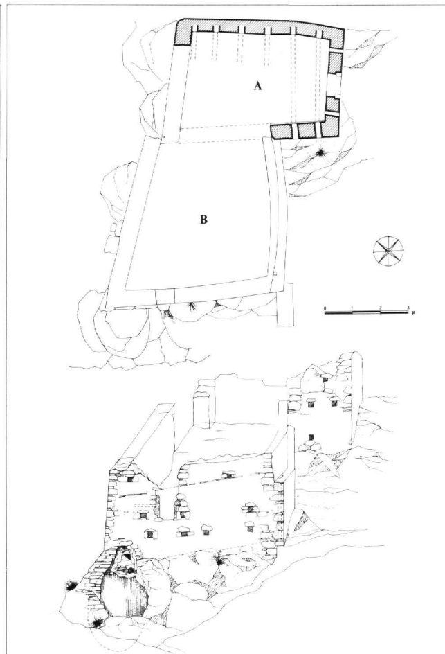
Εικ. 21. Κτίριο 16. Κάτοψη ανωγίου χώρου Α και δυτική εξωτερική όψη.
