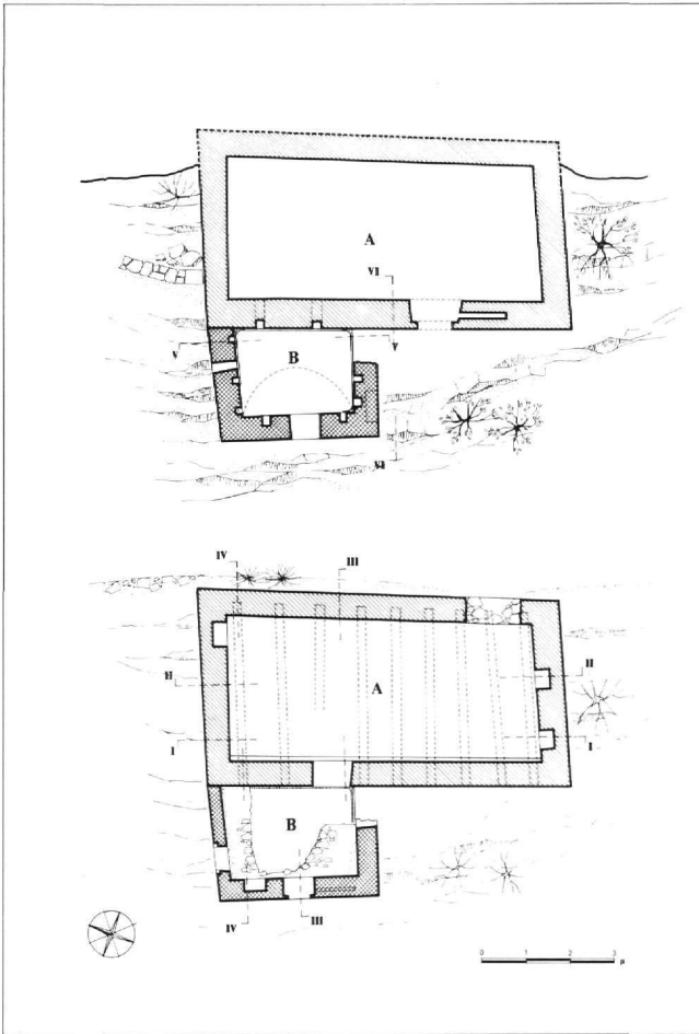
Εικ. 22. Κτίριο 13. Κάτοψη κατωγίων και ανωγίων.
