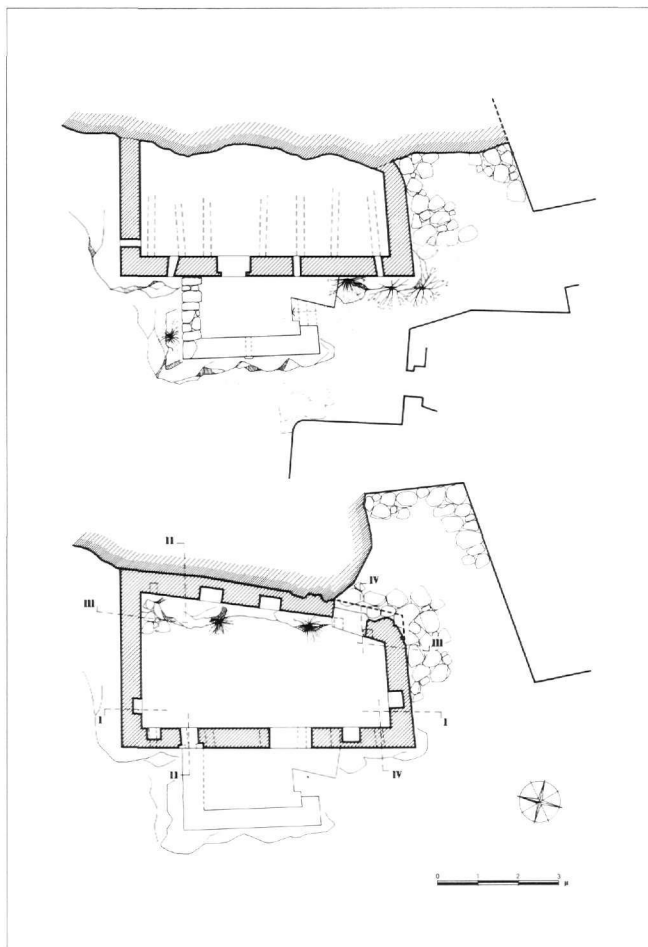
Εικ. 10. Κτίριο 8. Κάτοψη καταγίου και αναγίου.
