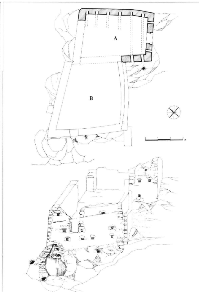
Εικ. 21. Κτίριο 16. Κάτοψη ανωγίου χώρου A και δυτική εξωτερική όψη.
