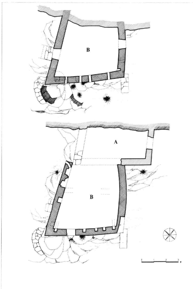
Εικ. 20. Κτίριο 16. Κάτοψη κατωγίου χώρου Β, ανωγίου χώρου Β και κατωγίου χώρου Α.
