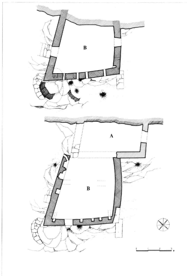
Εικ. 20. Κτίριο 16. Κάτοψη κατωγίου χώρου B, ανωγίου χώρου B και κατωγίου χώρου A.
