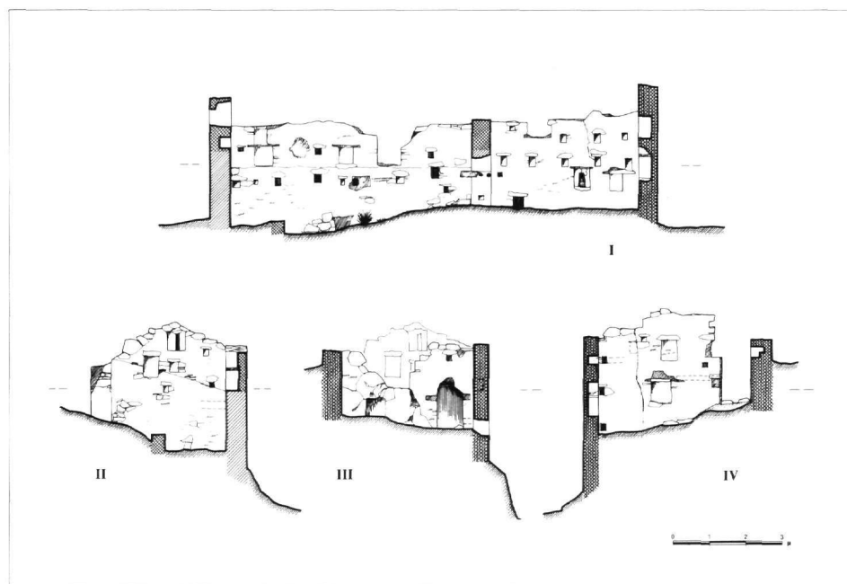
Εικ. 26. Κτίριο 14. Εξωτερική δυτική όψη, κάτοψη αναγίων και καταγίων.
