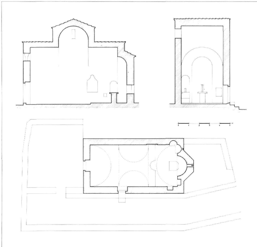
Εικ. 13. Ουζντινα Θεσπρωτίας. Ναός Ταξιαρχών. Κάτοψη και τομές.
