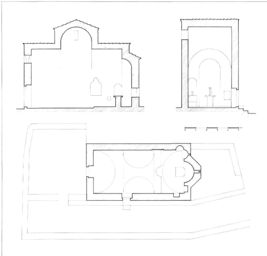
Εικ. 13. Ουζντινα Θεσπρωτίας. Ναός Ταξιάρχων. Κάτοψη και τομές.
