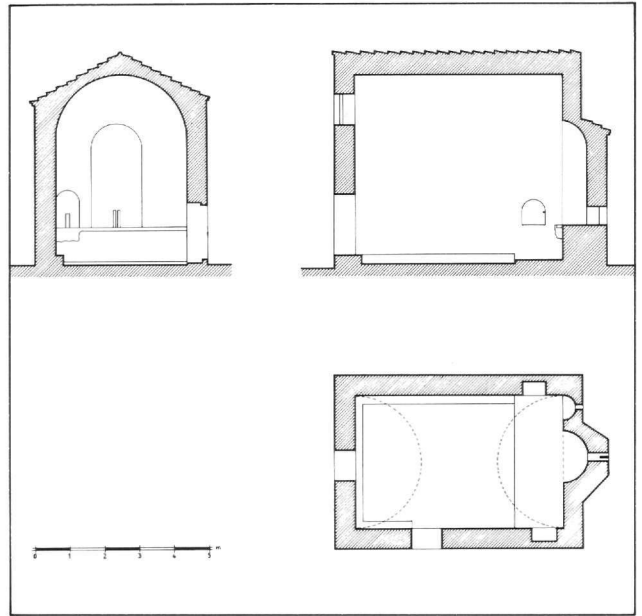
Εικ. 19. Ουζντίνα Θεσπρωτίας. Ναός Κοίμησης της Θεοτόκου. Κάτοψη και τομές.
