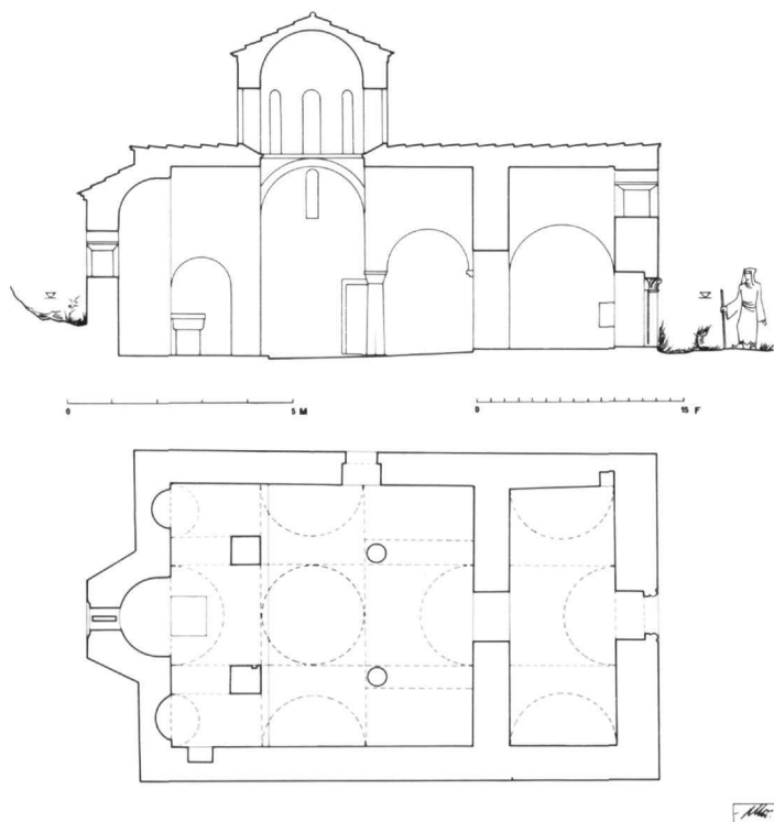
Εικ. 10. Ραχιώτισσα Φλιούντος. Κάτοψη και κατά μήκος τομή του ναού σε αποκατάσταση.
