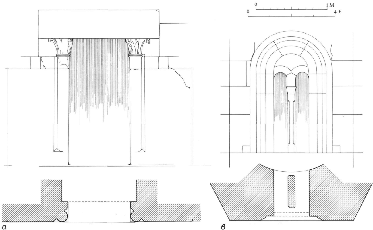
Είκ. 4. Ραχιώτισσα Φλιοῦντος: α. Ἡ δυτικὴ εἴσοδος (κάτοψη καὶ ὄψη), β. Τό παράθυρο τῆς κόγχης τοῦ Ἱεροῦ (κάτοψη καὶ ὄψη) σέ ἀναπαράσταση.
