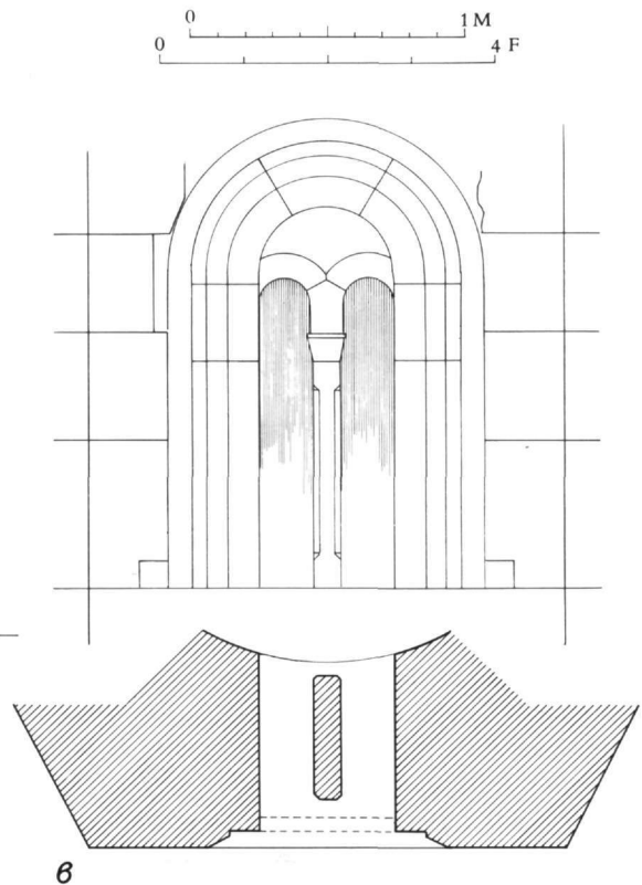
Είκ. 4. Ραχιώτισσα Φλιοῦντος: α. Ἡ δυτικὴ εἴσοδος (κάτοψη καὶ ὄψη), β. Τὸ παράθυρο τῆς κόγχης τοῦ Ἱεροῦ (κάτοψη καὶ ὄψη) σέ ἀναπαράσταση.
