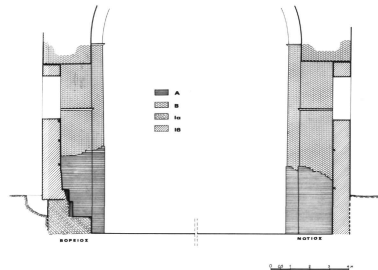
Εικ. 16. Εσωτερικό ανάπτυγμα της κόγχης του Ιερού: Α = Πρώτη παλαιοχριστιανική φάση. Β = Δεύτερη παλαιοχριστιανική φάση. Γ = Φάση 7ου αι.
