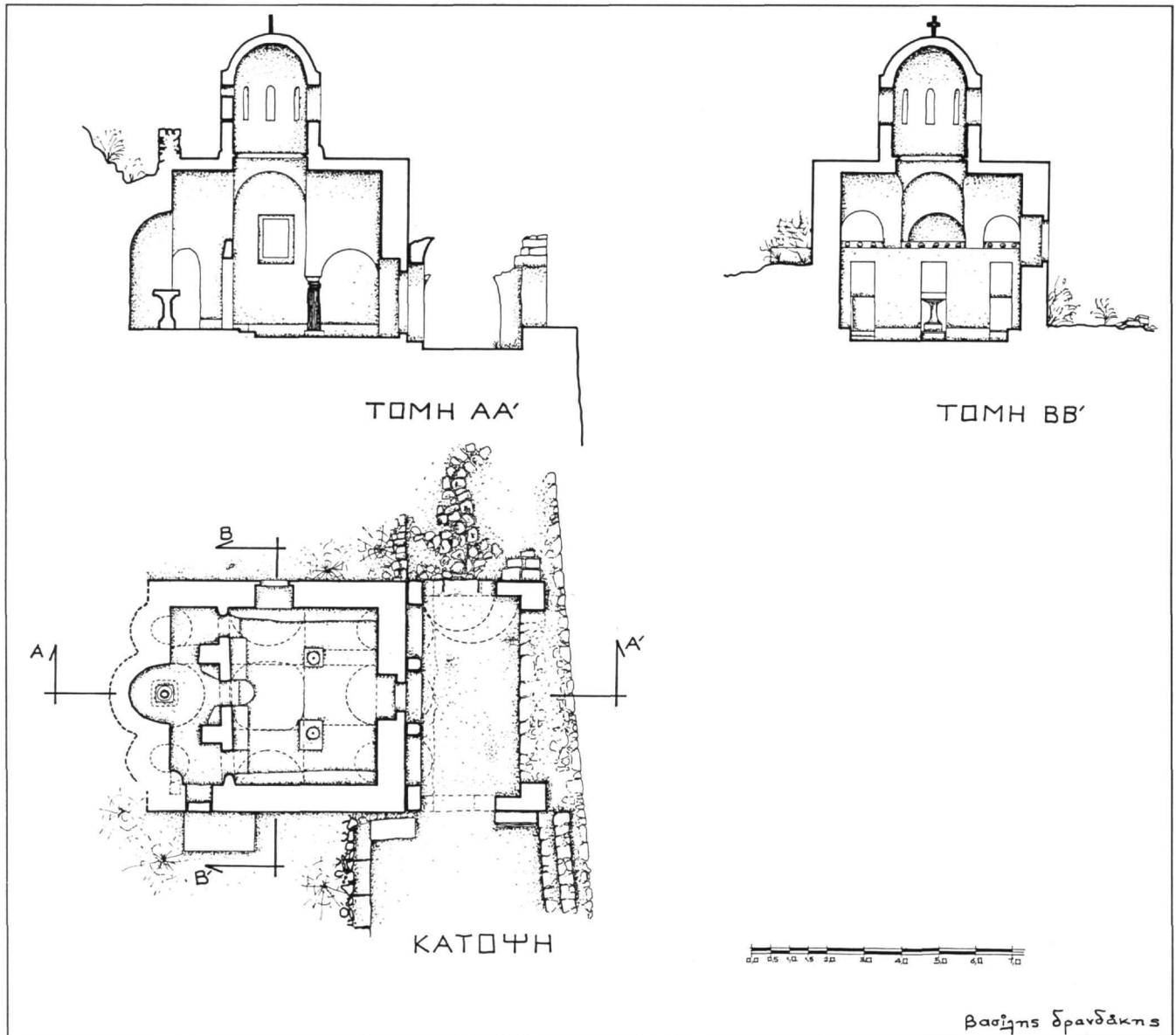
Εἰκ. 2. Κάτοψη καὶ τομές τοῦ Σωτήρα τοῦ Οἰτύλου.
