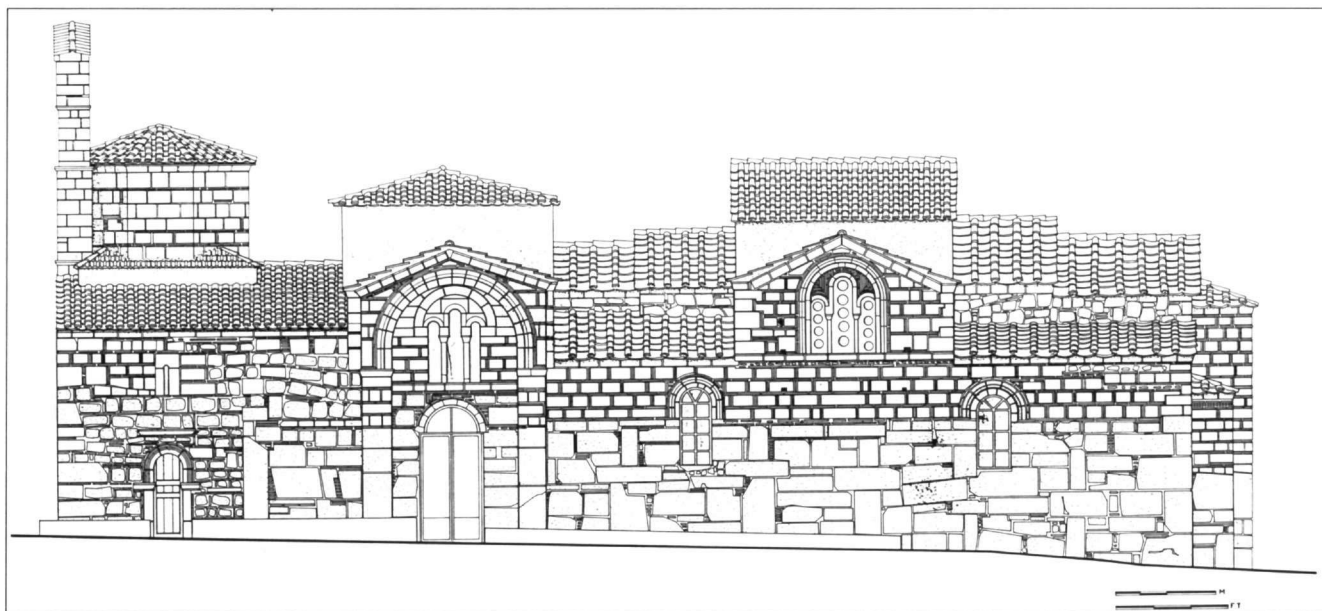
Εικ. 4. Μονή Σαγματά. Καθολικό. Νότια όψη.
