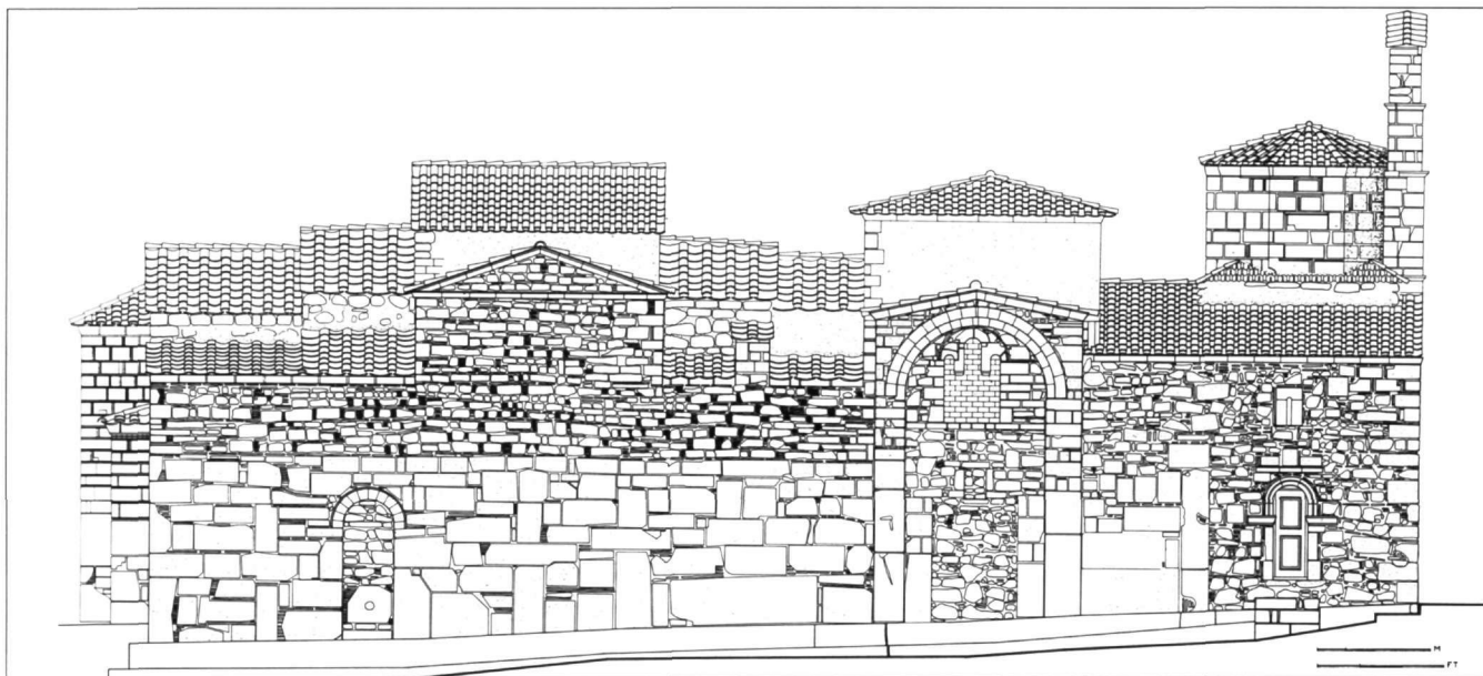
Εικ. 6. Μονή Σαγματά. Καθολικό. Βόρεια όψη.
