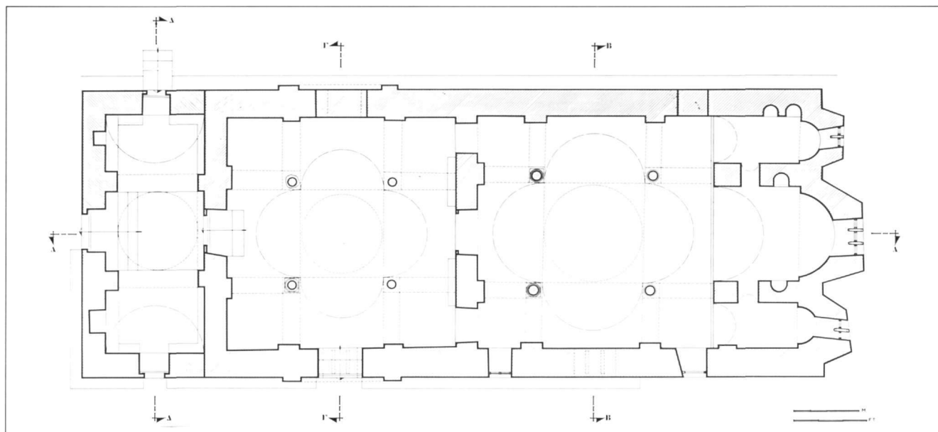
Ειγ. 2. Μονή Σαγματά. Καθολικό. Κάτοψη.
