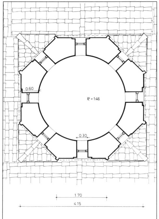
Εικ. 9. Μονή Σαγματά. Καθολικό. Γραφική αναπαράσταση της κάτοψης του τρούλου του κυρίως ναού.
