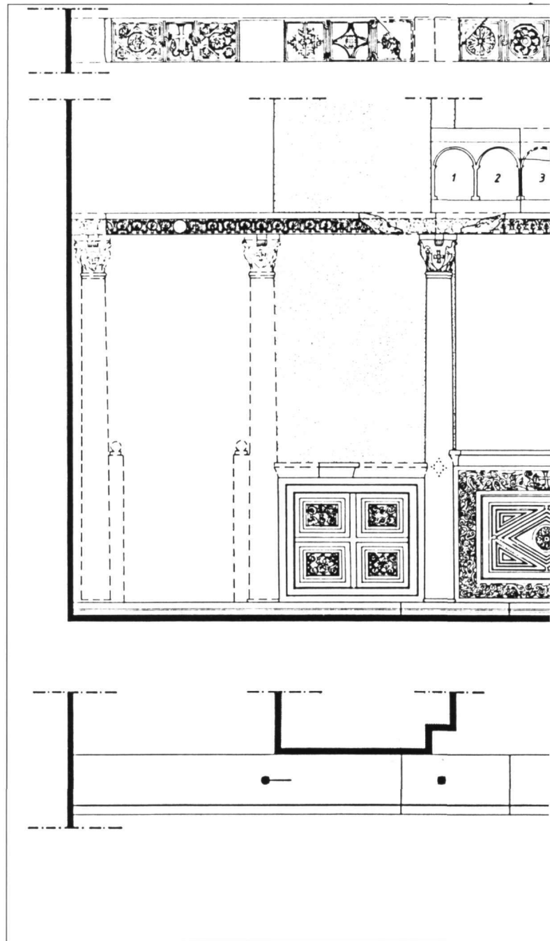
Εικ. 17. Καθολικό μονής Βατοπεδίου. Αναπαράσταση του μαρμαρίνου τέμπλου (όψη, άνοψη και τομή) και κάτοψη του στυλοβάτη στην υφιστάμενη κατάσταση.
