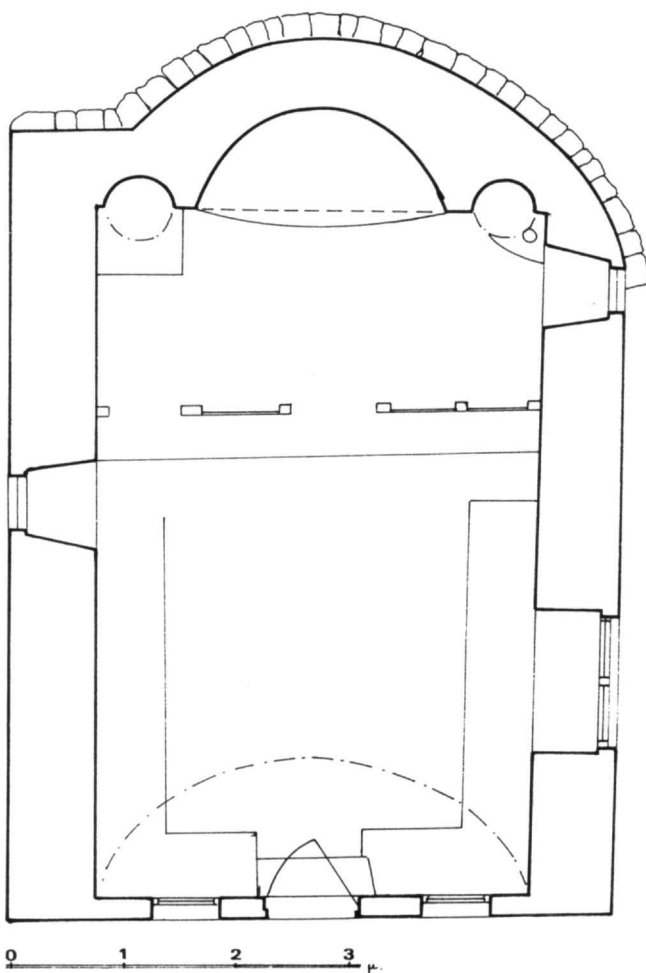
Εικ. 2. Ιερά Μονή Τιμίου Προδρομόν Σερρών. Προδρομοῦδι. Κάτοψη παρεκκλησίου.
