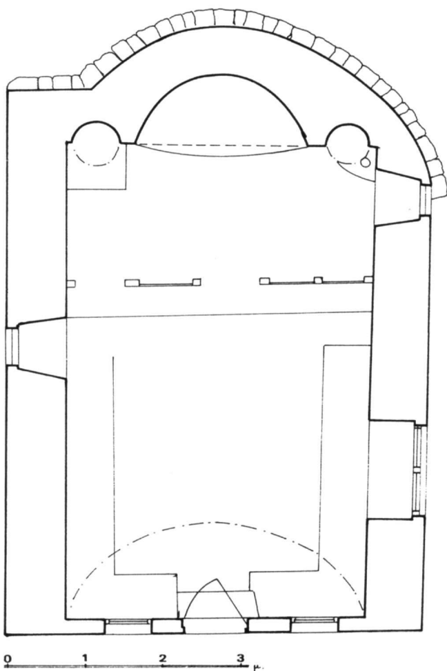
Εικ. 2. Ιερά Μονή Τιμίου Προδρόμου Σερρών. Προδρομούδι. Κάτοψη παρεκκλησίων.
