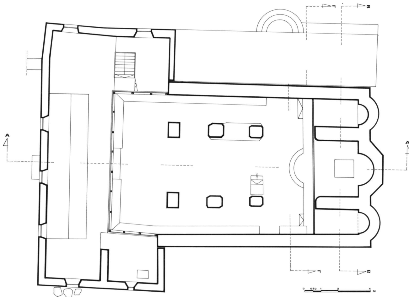
Εικ. 4. Μεγάλη Παναγιά. Κάτοψη γυναικωνίτη (υπόρχουσα κατάσταση).
