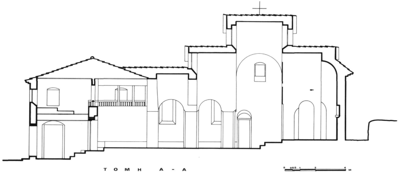
Εἰκ. 5. Μεγάλη Παναγιά. Τομή κατὰ μήκος (Α-Α) (ὑπάρχουσα κατάσταση).
