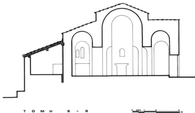
Εἰκ. 6-7. Μεγάλη Παναγιά. Ἐγκάρσιες τομές (Γ-Γ) καί (Β-Β) (ὑπάρχουσα κατάσταση).
