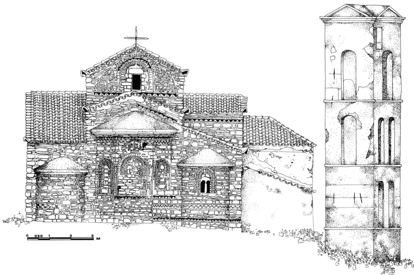
Εικ. 21. Μεγάλη Παναγιά. Ανατολική όψη του ναού (υπάρχουσα κατάσταση).
