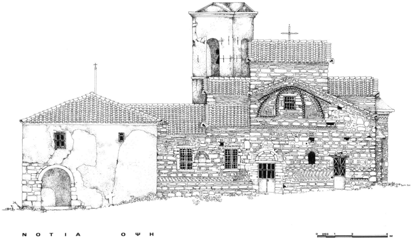
Εικ. 23. Μεγάλη Παναγιά. Νότια όψη του ναού (υπόχρονσα κατάσταση).
