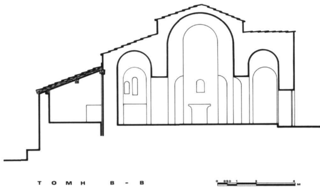
Εἰκ. 6-7. Μεγάλη Παναγιά. Ἐγκάρσιες τομές (Γ-Γ) καὶ (Β-Β) (ὑπάρχουσα κατάσταση).
