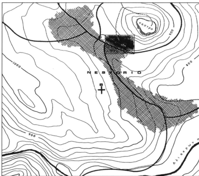
Εικ. 1. Νεστόριο. Τοπογραφικό διάγραμμα.
