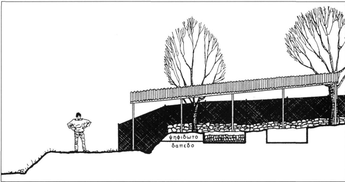
Εικ. 2. Κάστρο Νεστορίου. Τομή της ανασκαφής.
