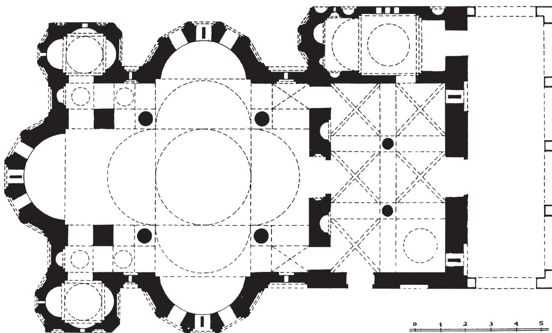
Εικ. 3. Καθολικόν Μονής Αντινίτσης (Ορλάνδος). Λιτή με ενιαία κάλυψη μονώροφη.
