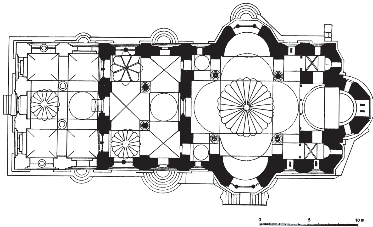
Εικ 7. Καθολικόν Χελανδαρίου, Άγιον Όρος (Nenadovic).
