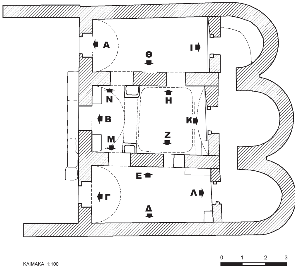
Εικ. 1. Καμπινάρι, Πλάτσα. Άγιος Νικόλαος. Κάτοψη.
