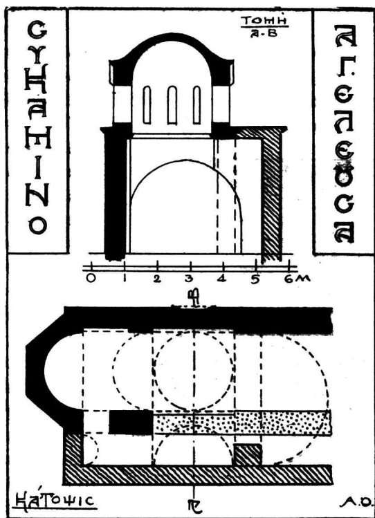
Εἰκ. 17. Κάτοψις καὶ κατὰ πλάτος τομὴ ναοῦ Ἀγ. Ἐλεούσης ἐν Συκαμίνῳ.
