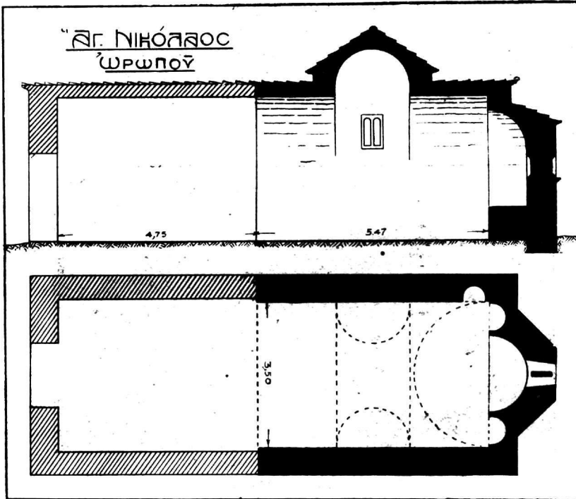
Εἰκ. 14. Κάτοπις καὶ τομὴ ναοῦ Ἁγίου Νικολάου Ὁρωποῦ.
