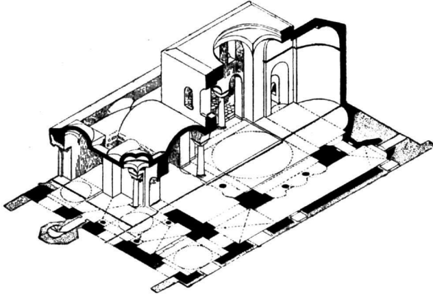
Εἰκ. 20. Ναὸς Ἁγίου Ἀνδρέου ἐν τῇ Κρῖσει. Κλ. 1:500.
